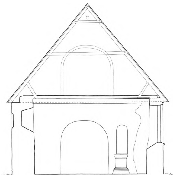
Fig. 5. Tværnsnit 1:150 gennem skib, set mod øst. Målt af Henrik Jacobsen 1984, tegnet af Marianne Nielsen 1992. – Querschnitt durch Schiff gegen Osten .
