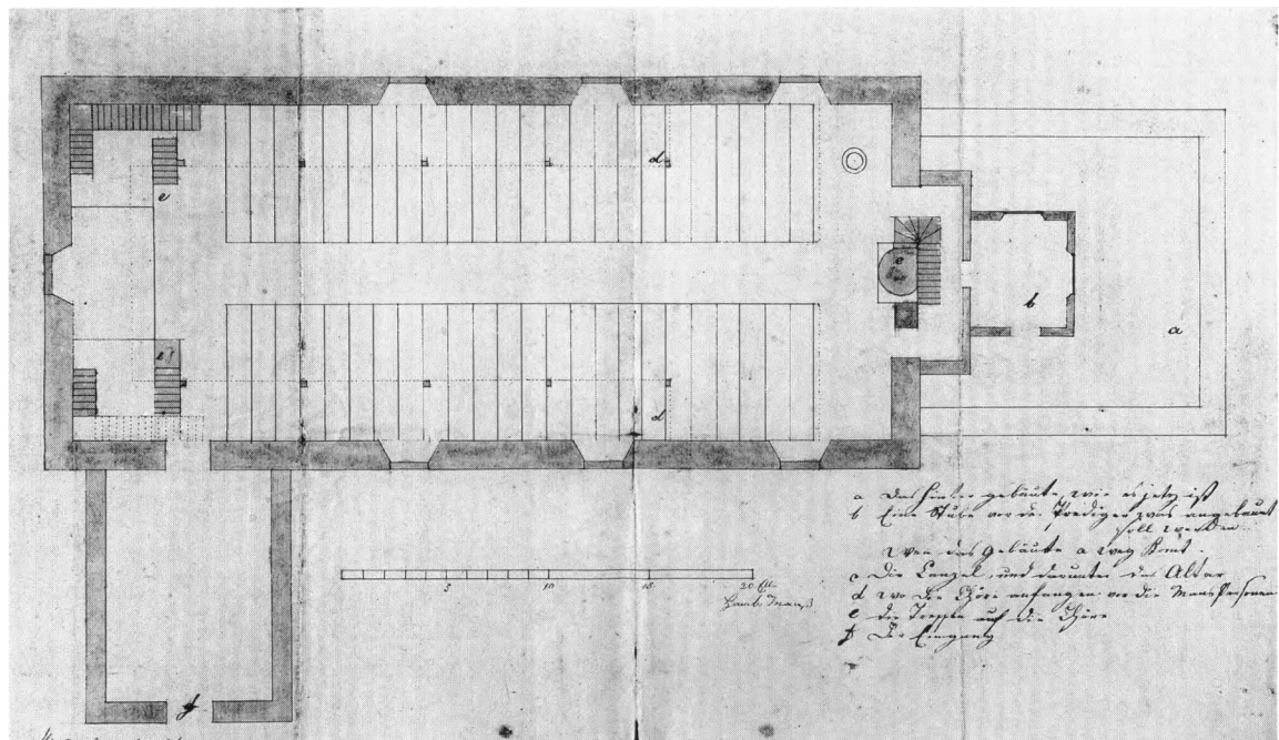
Fig. 27. Grundplan af kirken med forslag til ombygning og nyindretning, 1797 (s. 2648). a. Det romanske kor, foreslået nedrevet, b. Forslag til »præsteværelse« (sakristi), c. Prædikestolsalter (s. 2654, 2661). d. Pulpiturer. e. Trappe til pulpitur, f. Våbenhusdør. Mål i hamborgske alen. Tegning med tysk tekst i Landsarkivet for Nørrejylland. – Grundriss von der Kirche mit Vorschlägen für Umbau und Neueinrichtung , 1797. a. Romanischer Chor (Abbruch vorgeschlagen), b. Vorschlag für »Pfarrzimmer« (Sakristei), c. Kanzelaltar, d. Emporen, e. Treppe zur Empore, f. Eingang zum Vorhaus. Massangaben in hamburgischen Ellen. Zeichnung bei dem Landesarchiv für Nørrejylland.
