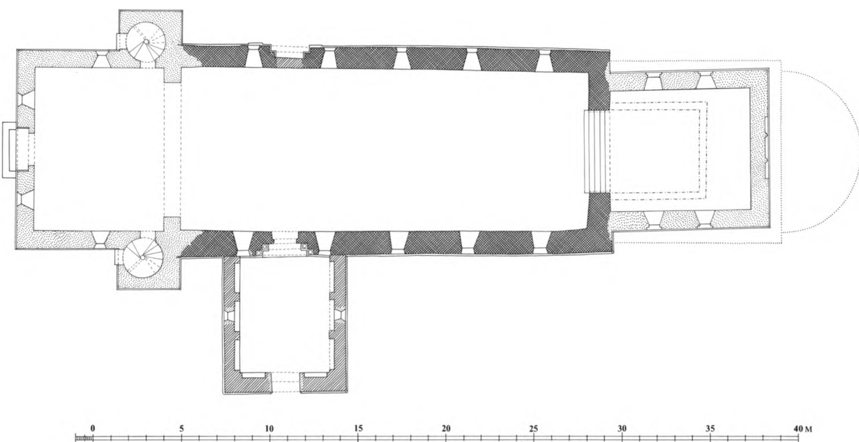
Fig. 4. Grundplan 1:300, målt af Henrik Jacobsen og Marianne Nielsen 1986, tegnet af sidstnævnte 1992. Den punkterede linie angiver det romanske \dagger kor med apsis, stiplingen \dagger sakristiet 1797-1919. – Grundriss. Die gepunktete Linie zeigt den romanischen \dagger Chor mit Apsis an, die gestrichelte Linie die \dagger Sakristei, 1797-1919.
