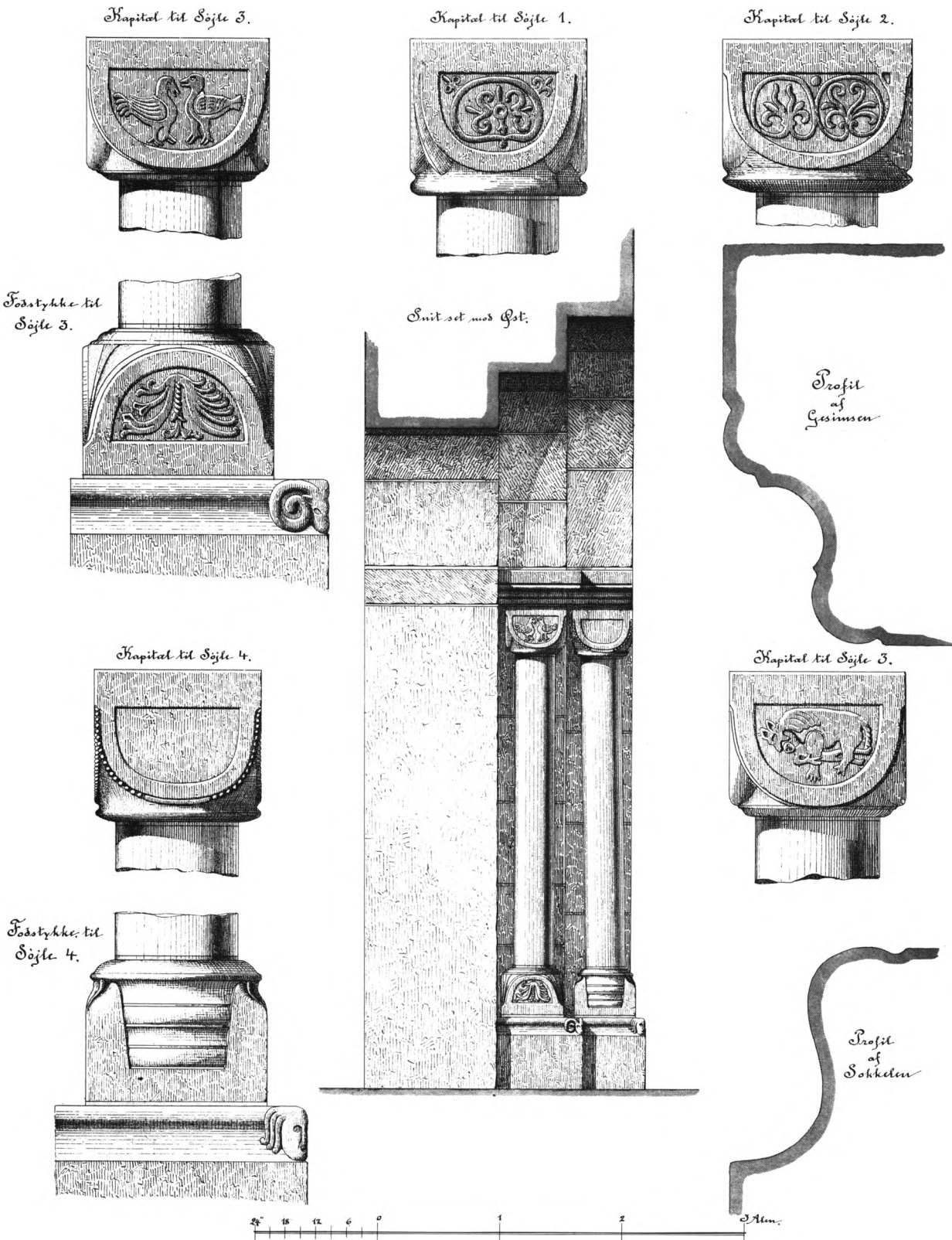
Fig. 10. Sydportal. Snit set mod øst 1:30 samt detaljer af kapitæler og baser (s. 2636). Målt og tegnet af F. Uldall 1888. – Das Südportal. Schnitt gegen Osten sowie Details von Kapitellen und Basen. Vermessen 1888.
