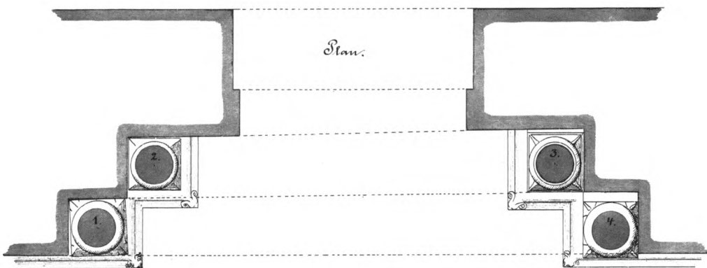
Fig.9. Sydportal. Opstalt og plan 1:30 (s. 2635). Målt og tegnet af F. Uldall 1888. — Das Südportal. Aufriss und Grundriss, vermessen 1888.
