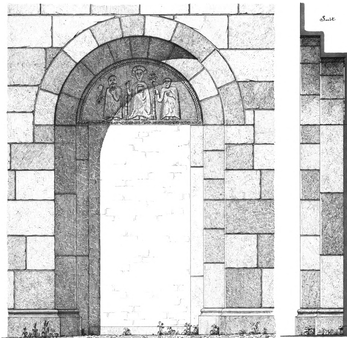
Fig. 15. Norddør. Opstalt og snit mod øst 1:30 (s. 2636). Målt og tegnet af F. Uldall 1888. – Das Nordportal. Aufriss und Schnitt gegen Osten. Vermessen 1888.
