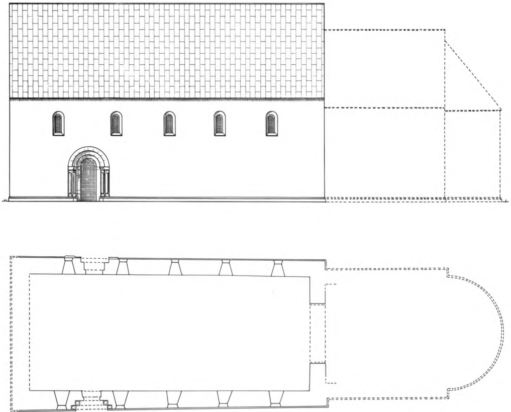
Fig. 7-8. Rekonstruktion af det romanske anlæg. 7. Opstalt. 8. Grundplan. 1:300, tegnet af Marianne Nielsen efter udkast af Niels Jørgen Poulsen 1992. – Rekonstruktion der romanischen Anlage. Aufriss und Grundriss.
