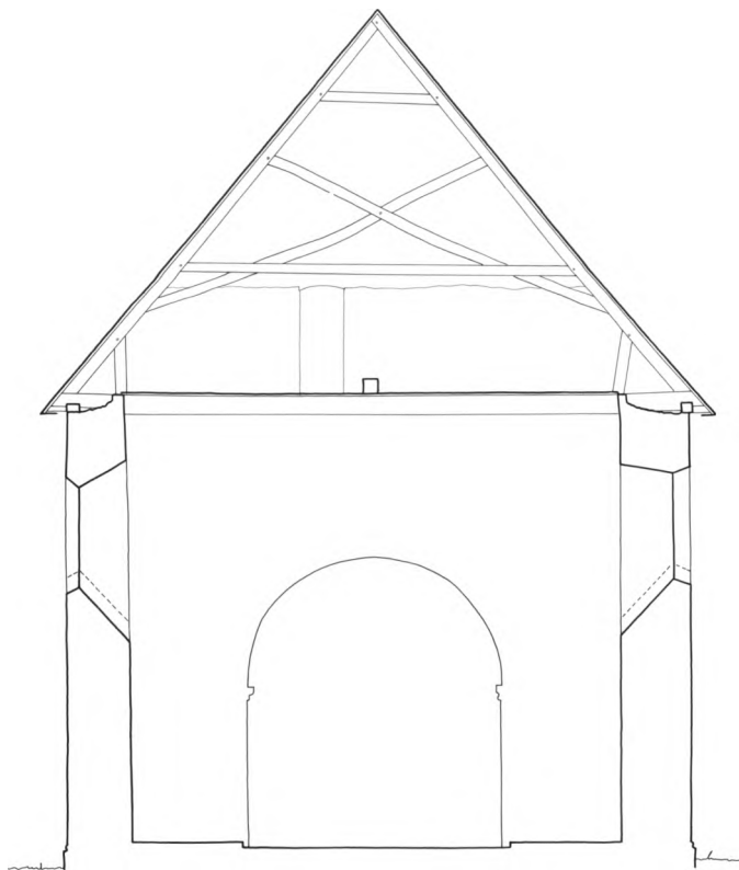
Fig. 6. Tværnsnit 1:150 gennem skibet, set mod øst. Målt af Henrik Jacobsen og Marianne Nielsen 1986, tegnet af sidstnævnte 1992. – Querschnitt durch Schiff gegen Osten.
