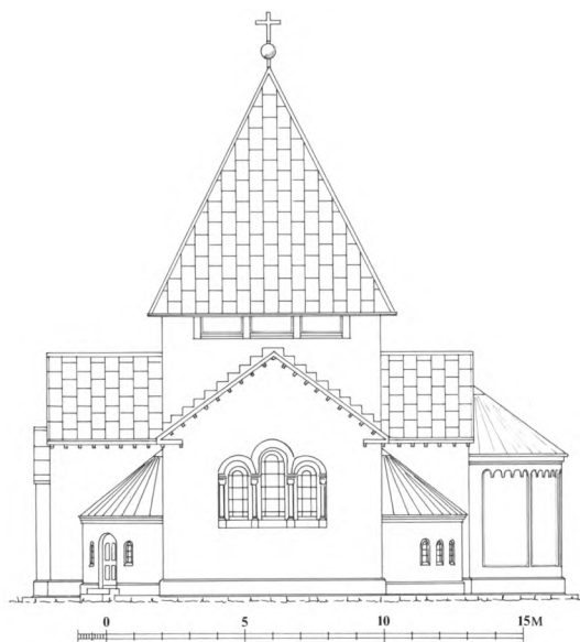
Fig. 3-4. Grundplan og opstalt af kirken set fra syd. 1:300. Efter forslag til ombygning ved Richard Aas 1964, i Lokallhistorisk Arkiv for Holsted kommune. Tegnet af Marianne Nielsen 1993. – Grundriss und Aufriss der Kirche, Südansicht.
