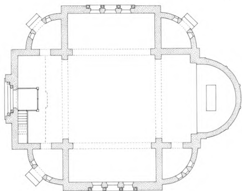
Fig. 3-4. Grundplan og opstalt af kirken set fra syd. 1:300. Efter forslag til ombygning ved Richard Aas 1964, i Lokallhistorisk Arkiv for Holsted kommune. Tegnet af Marianne Nielsen 1993. – Grundriss und Aufriss der Kirche, Südansicht.
