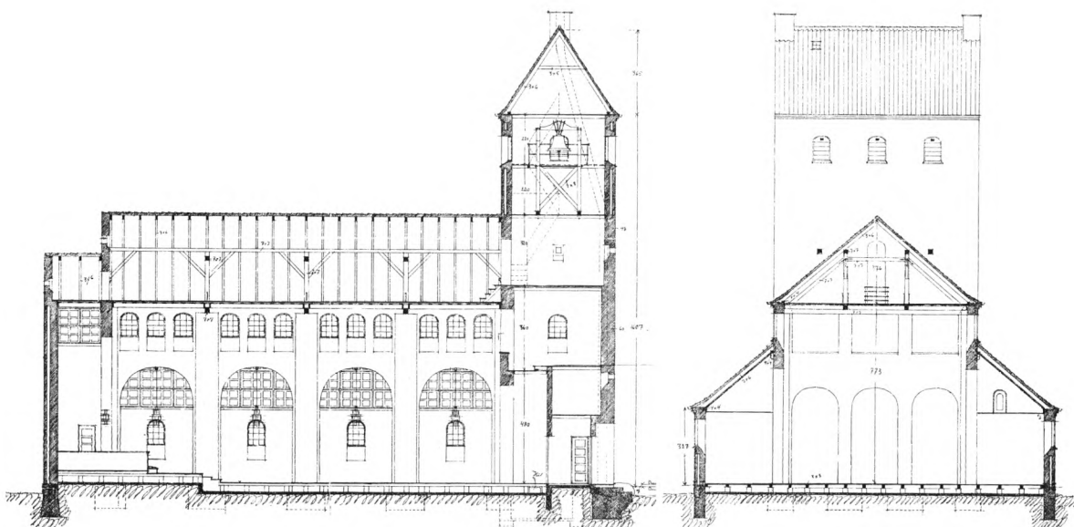
Fig. 4-5. Længdesnit set mod syd og tværsnit mod vest ved Rolf Schroeder 1924. 1:300. Ved embedet. – Längsschnitt gegen Süden und Querschnitt gegen Westen, 1924.
