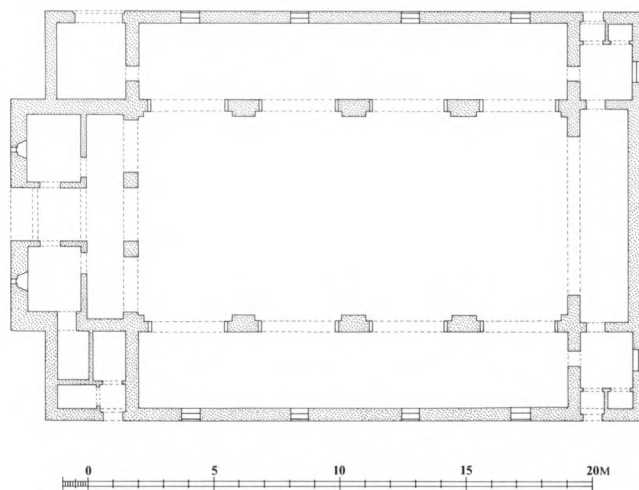
Fig. 2. Grundplan 1:300, målt af Henrik Jacobsen og tegnet af Marianne Nielsen 1993. – Grundriss.
