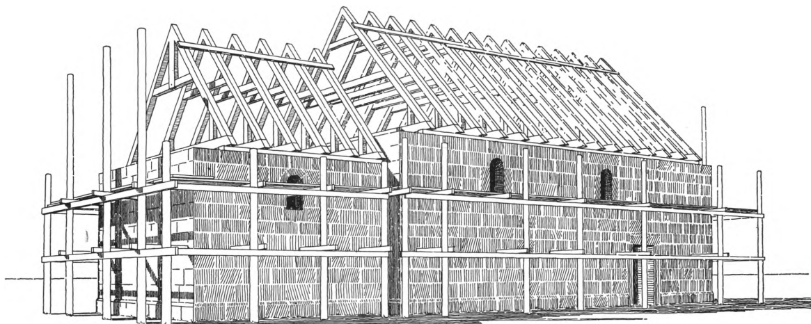
Fig. 7. Kirken under opførelse. Rekonstruktionsforslag ved Knud J. Krogh (s. 2807). Efter Aarbøger for nordisk Oldkyndighed 1959. – Die Kirche während des Baus. Vorschlag zur Rekonstruktion.
