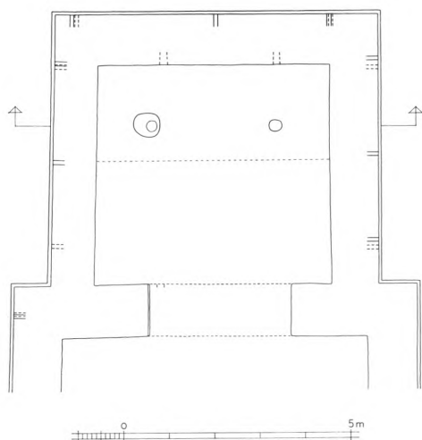
Fig. 8. Arkæologiske undersøgelser i koret 1958. Plan og tværsnit set mod øst 1:150. Jordlagene er angivet med tal: 1. oprindelig terræn, 2. og 3. afretningslag, 4. byggelag. Bevarede bomhuller i murens yderside er indtegnet (i 4. skifte med fuld streg, i 8. skifte med punkteret streg) og byggestilladserne er søgt rekonstrueret (s. 2807). Tegnet af Knud J. Krogh. Efter Aarbøger for nordisk Oldkyndighed 1959. – Archäologische Untersuchungen im Chor 1958. Grundriss und Querschnitt gegen Osten. Die Zahlen weisen auf die Erdschichten hin: 1. Gewachsener Boden, 2. und 3. Ausgleichschichten, 4. Bauschicht. Die erhaltenen Rüstlöcher an der Aussenseite der Mauern sind eingezeichnet (in 4. Schicht mit einer ungebrochenen Linie, in 8. Schicht mit einer gestrichelten Linie). Die Baugerüste versuchsweise rekonstruiert.
