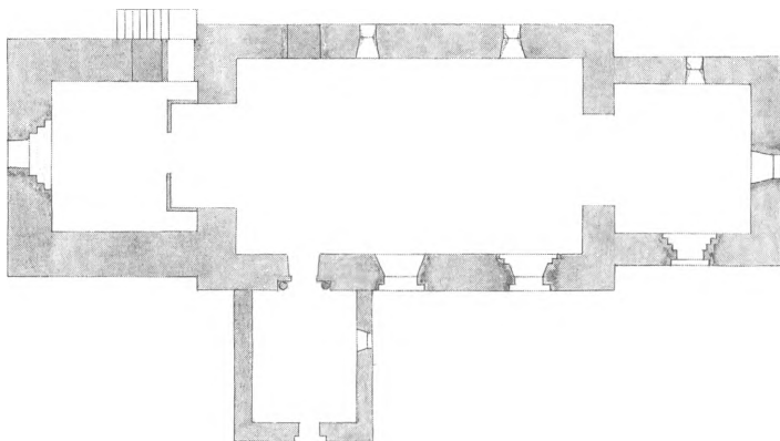
Fig. 13. Grundplan af kirken 1:300, målt i forbindelse med herredsrejse (1875). – Grundriß, vermessen 1875.
