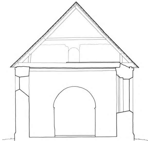
Fig. 6. Tværsnit 1:150 gennem skib, set mod øst. Målt af Henrik Jacobsen og tegnet af Marianne Nielsen 1993. – Querschnitt durch Schiff gegen Osten.
