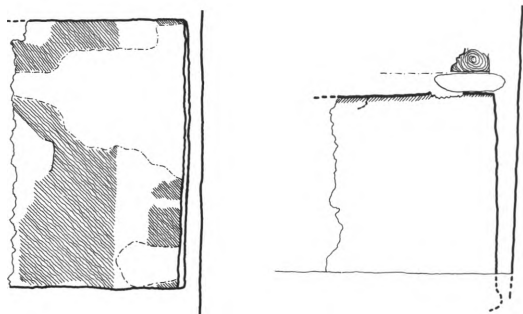
Fig. 17. Alterbord, romansk, muret af hele og kløvede marksten, reduceret ved forhugning fortil 1870 (s. 2816). Bordfladen har rester af en helgengrav og ca. 20 cm fra bagkanten spor efter en trinagtig forhøjning, som må have været støtte for et samtidigt, kobberklædt retabel (s. 2822, jfr. fig. 18 og 26). Plan og snit, 1:50, ved Knud J. Krogh 1971. – Romanischer Altartisch aus Feldstein, 1870 reduziert an der Vorderseite. In der Altartischplatte befinden sich Reste eines Sepulcrums. Etwa 20 cm von der Hinterkante gibt es Spuren einer stufenartigen Erhöhung, die als Stütze eines gleichzeitigen, kupfergedeckten Retabels gedient haben mag (vgl. Abb. 18 und 26).
