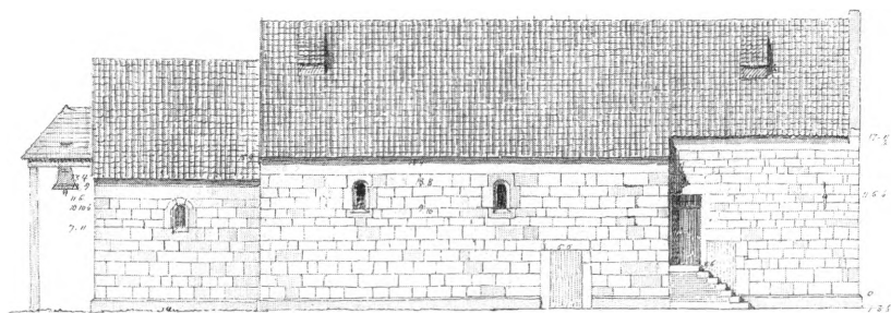
Fig. 12. Opstalt af kirkens nordside 1:300, målt i forbindelse med herredsrejse (1875). – Aufriß, Nordseite der Kirche, vermessen 1875.
