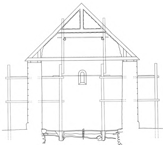
Fig. 8. Arkæologiske undersøgelser i koret 1958. Plan og tværsnit set mod øst 1:150. Jordlagene er angivet med tal: 1. oprindelig terræn, 2. og 3. afretningslag, 4. byggelag. Bevarede bomhuller i murens yderside er indtegnet (i 4. skifte med fuld streg, i 8. skifte med punkteret streg) og byggestilladserne er søgt rekonstrueret (s. 2807). Tegnet af Knud J. Krogh. Efter Aarbøger for nordisk Oldkyndighed 1959. – Archäologische Untersuchungen im Chor 1958. Grundriss und Querschnitt gegen Osten. Die Zahlen weisen auf die Erdschichten hin: 1. Gewachsener Boden, 2. und 3. Ausgleichschichten, 4. Bauschicht. Die erhaltenen Rüstlöcher an der Aussenseite der Mauern sind eingezeichnet (in 4. Schicht mit einer ungebrochenen Linie, in 8. Schicht mit einer gestrichelten Linie). Die Baugerüste versuchsweise rekonstruiert.
