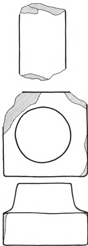
Fig. 46. Søjlefragmenter af granit, nu på loftet (s. 2813). Målt af NJP og tegnet af MN 1993. 1:10 – Säulenfragmente aus Granit, heute abgestellt.
