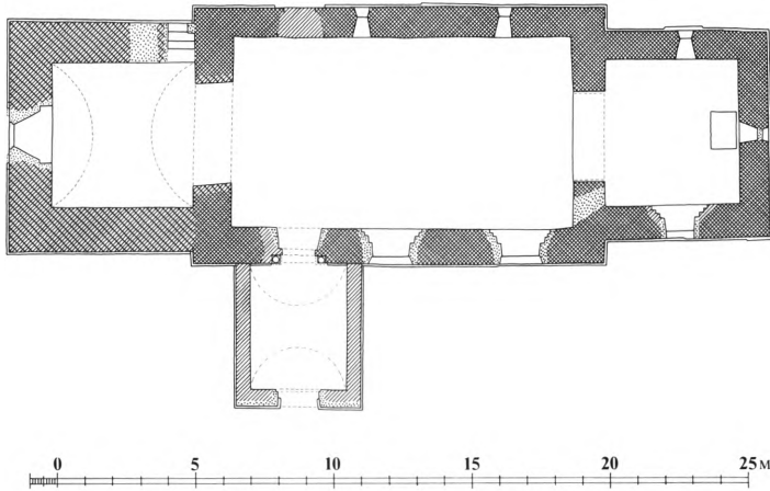
Fig. 5. Grundplan 1:300. Målt af Henrik Jacobsen og tegnet af Marianne Nielsen 1993. – Grundriss.
