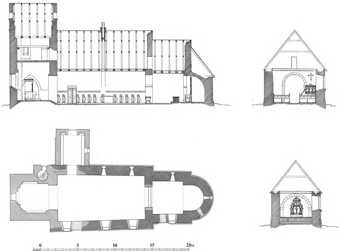
Fig. 4. Grundplan og snit, 1:300, målt af Aage Bugge og Rudolph Gram 1946. Grundplanen omtegnet af Marianne Nielsen 1993. – Grundriss .
