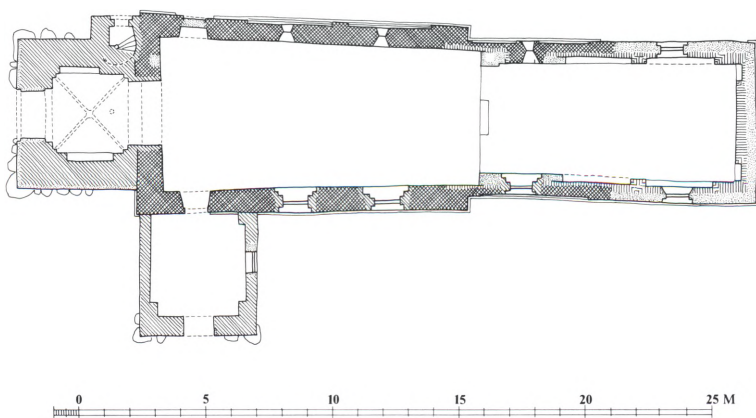
Fig. 4. Grundplan 1:300. Målt af HeJ 1977 og tegnet af Mogens Vedsø 1995. – Grundriß .
