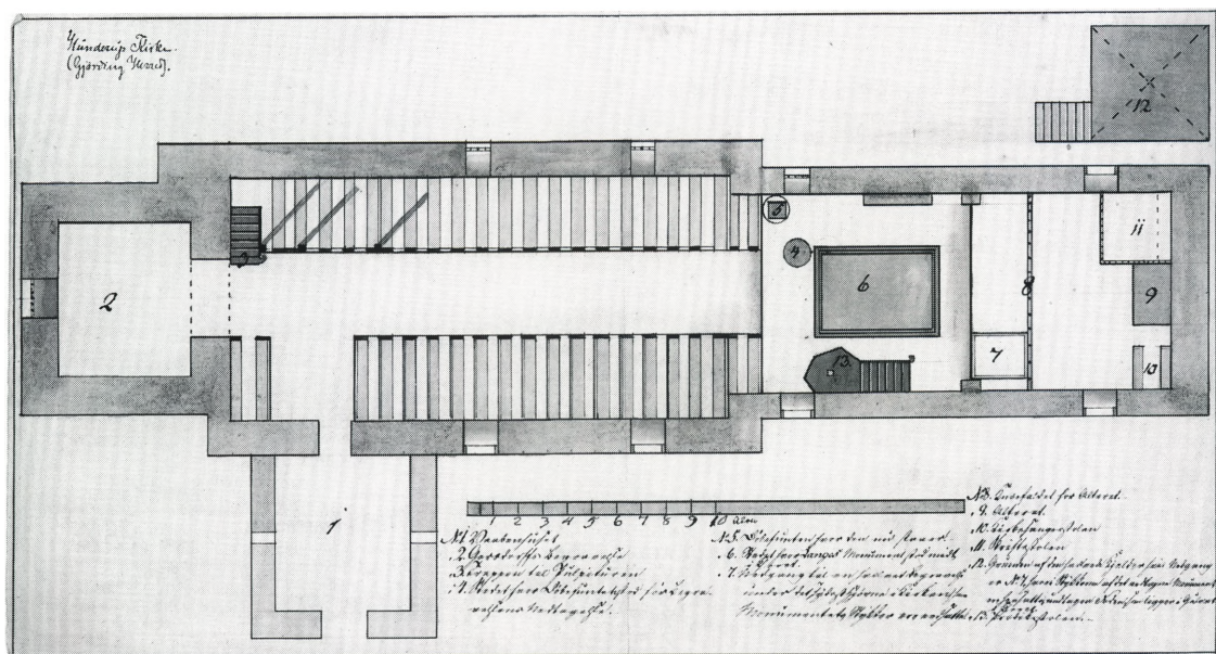
Fig. 9. Indretningsplan 1822. De anførte tal angiver ifølge påskriften: 1. Våbenhuset. 2. Gersdorffs begravelse. 3. Trappen til pulpituret. 4. Stedet hvor døbefonten stod før begravnens nedtagelse. 5. Døbefonten hvor den nu står. 6. Stedet hvor Langes monument stod midt i koret. 7. Indgang til en hvælvet begravelse under det sydøstre hjørne i kirken, hvor monumentets stykker er nedsatte. 8. Knæfaldet for alteret. 9. Alteret. 10. Kirkesangerstolen. 11. Skriftestolen. 12. Grunden af den hvælvede kælder, hvis nedgang er nr. 7, hvori stykkerne af det nedtagne monument er hensatte undtagen siden, som ligger i gulvet. 13. Prædikestolen. Tegning, måske ved Jeppe Stavn. – Einrichtungsplan 1822. Laut Beschriftung zeigen die angegebenen Zahlen folgendes an: 1. Vorhaus. 2. Begräbnis Gersdorffs. 3. Treppe zur Empore. 4. Lage der Taufe vor der Beseitigung des Begräbnisses. 5. Heutige Lage der Taufe. 6. Die ehemalige Lage des Grabmal Langes mitten im Chor. 7. Eingang zu einer Gruft unter der südöstlichen Ecke in der Kirche, wo die Einzelteile vom Monument aufbewahrt werden. 8. Betschemel vor dem Altar. 9. Der Altar. 10. Der Kirchensängerstuhl. 11. Der Beichtstuhl. 12. Der Grund des gewölbten Kellers, dessen Niedergang Nr. 7 ist, und wo die Einzelteile vom abgerissenen Monument abgestellt sind, abgesehen vom Seitenstück, der im Fußboden liegt. 13. Der Kanzel. Zeichnung, vielleicht von Jeppe Stavn.
