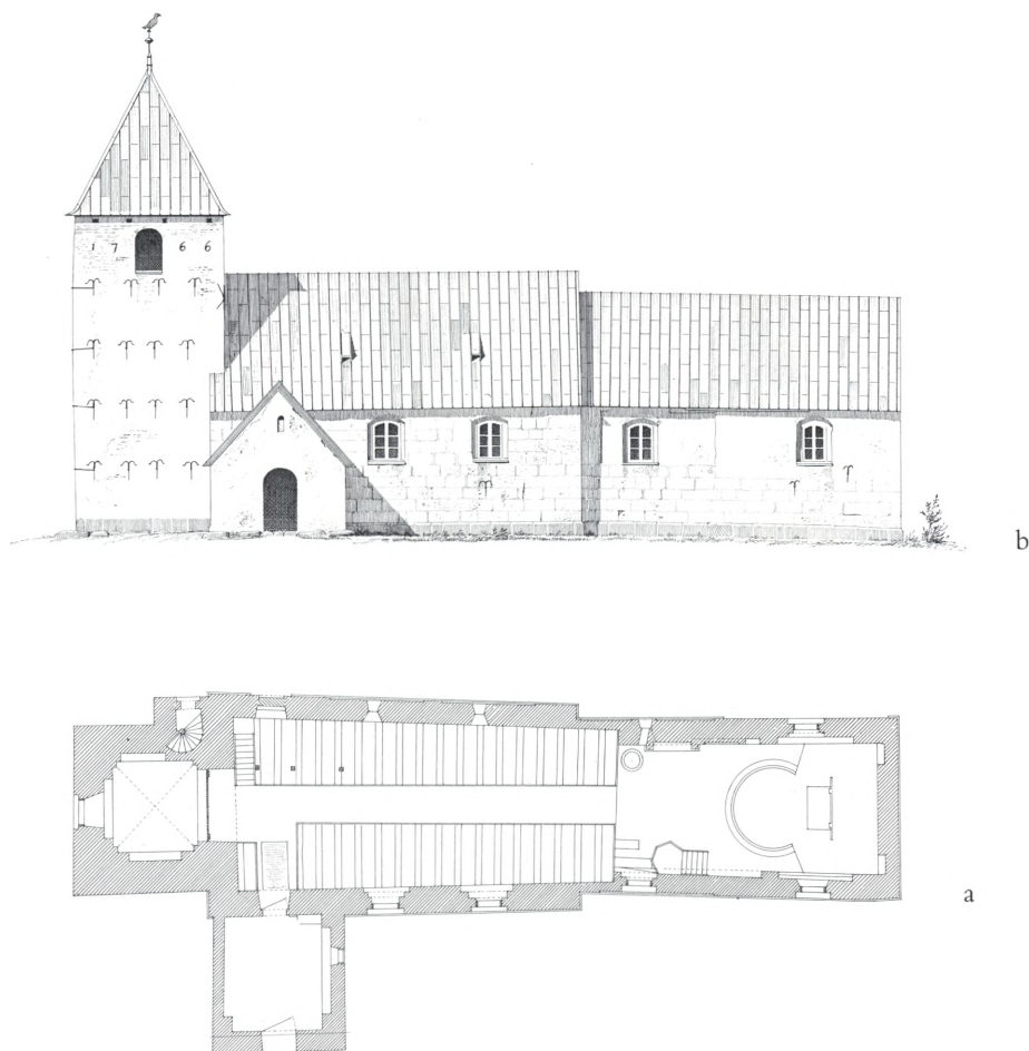
Fig. 6a-e. Opmålinger 1:300. a. Plan. b. Opstalt af kirkens sydside. c. Opstalt af kirkens nordside. d. Opstalt af kirkens østside. e. Tværsnit af kirken set mod øst. Forlæg til Danske Tufstenskirker. Målt og tegnet af V. Koch 1885. — a. Grundriß. b. Aufriß, Südwall der Kirche. c. Aufriß, Nordwall der Kirche. d. Aufriß, Ostwall der Kirche. e. Querschnitt. 1885.
