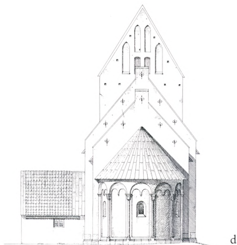
Fig. 7a-d. Opmålinger 1:300. a. Plan. b. Opstalt af sydsiden. c. Opstalt af nordsiden. d. Opstalt af østsiden. Forlæg til Danske Tufstenskirker. Målt og tegnet af Erik Schiødt 1884. – a. Grundriß. b. Aufriß von Südseite. c. Aufriß von Nordseite. d. Aufriß von Ostseite. Vermessen 1884.
