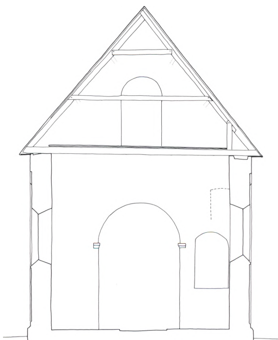
Fig. 5. Tværsnit 1:150. Målt af HeJ 1977 og tegnet af Mogens Vedsø 1995. – Querschnitt .
