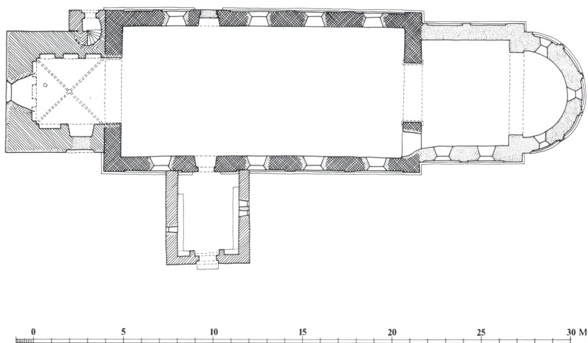
Fig. 4. Plan 1:300. Målt af HeJ 1977 og tegnet af Mogens Vedsø 1995. – Grundriß .
