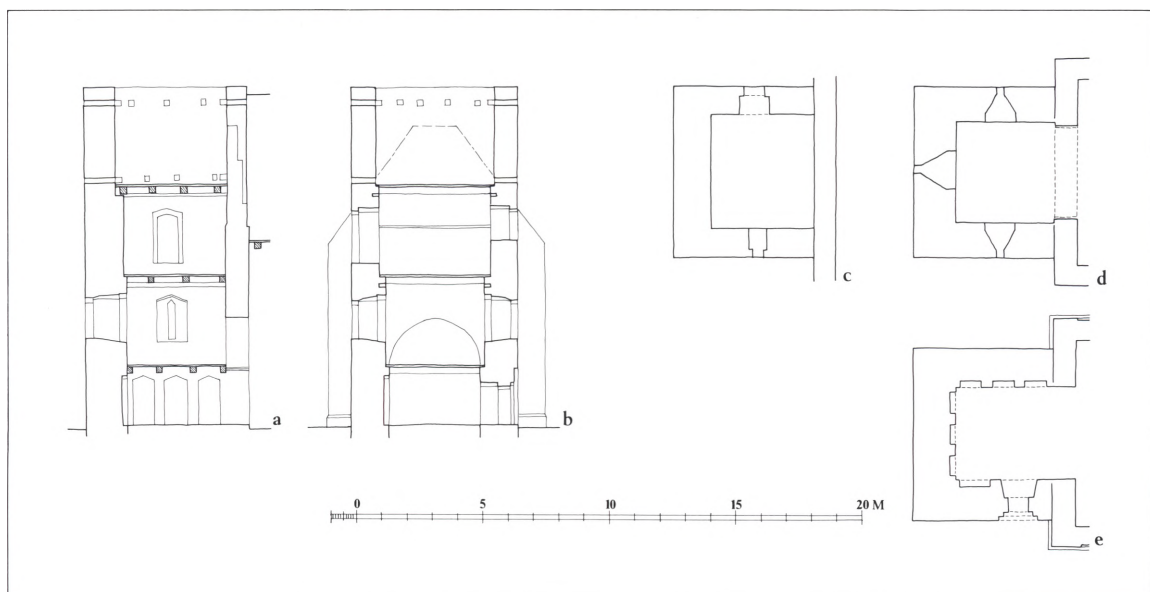
Fig. 13. Rekonstruktionsskitser af tårnet i oprindelig skikkelse 1:300. a. Snit set mod nord. b. Snit set mod øst. c. Plan af mellemstokværket. d. Plan af tårnrummet i højde med vinduerne. e. Gulvplan af tårnrummet. Målt og tegnet af Mogens Vedsø 1995. – Rekonstruktionsskizzen vom Turm in seiner ursprünglichen Gestalt. a. Schnitt gegen Norden. b. Schnitt gegen Osten. c. Plan vom Zwischenstockwerk. d. Plan vom Turmraum, Fensterhöhe. e. Bodenplan vom Turmraum.
