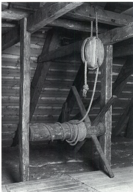
Fig. 15. Vinde på skibets loft (s. 3223). NE fot. 1994. - Winde auf Schiffsdachboden.
