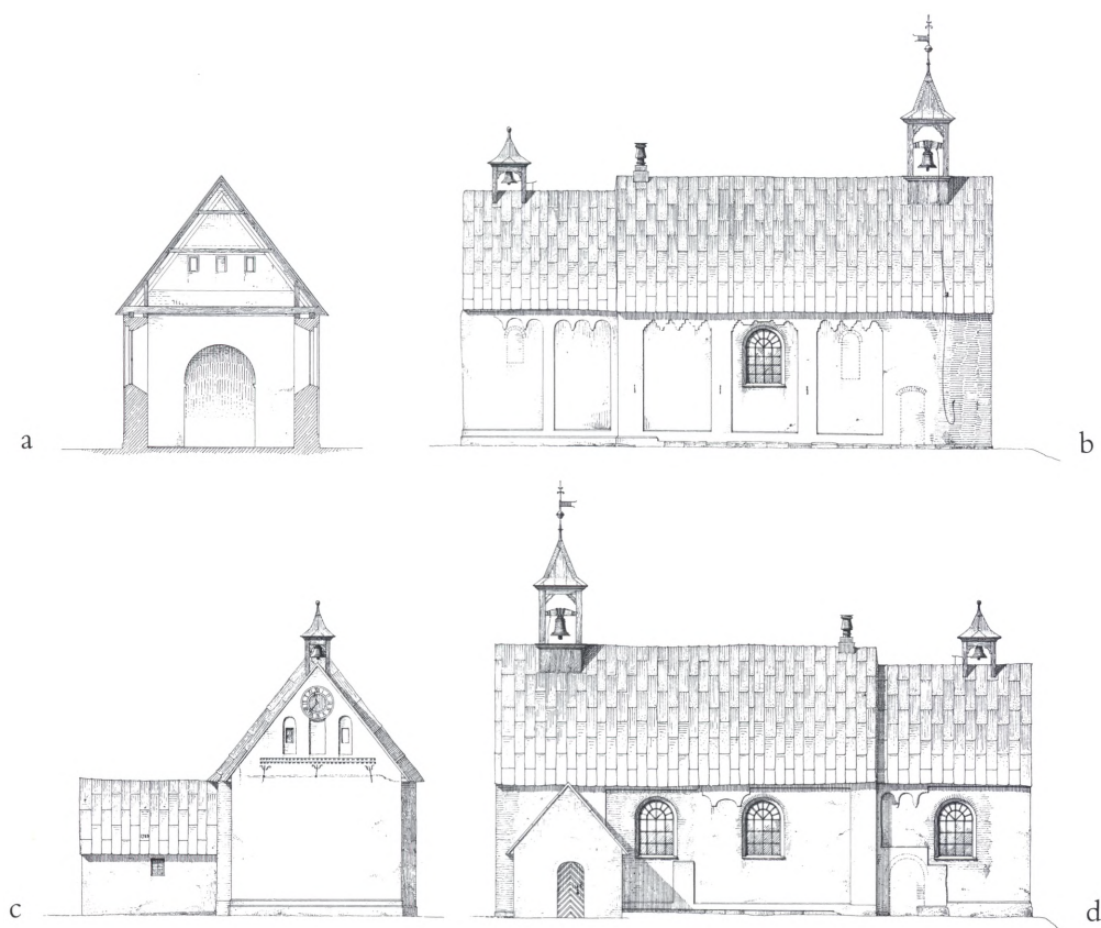
Fig. 5a-d. Opmålinger 1:300. a. Tværsnit af kirken set mod øst. b. Opstalt af kirkens nordside. c. Opstalt af kirkens østside. d. Opstalt af kirkens sydside. Forlæg til Danske Tufstenskirker. Målt og tegnet af E. Schiøtte 1884. – a. Querschnitt gegen Osten . b. Aufriß, Nordwand der Kirche . c. Aufriß, Ostwand der Kirche . d. Aufriß, Südwand der Kirche . 1884.
