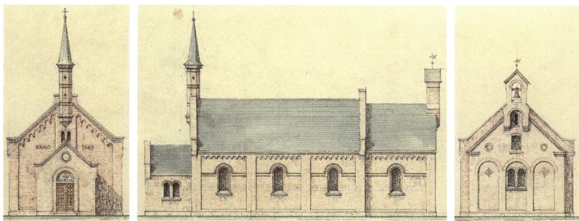
Fig. 2. Opstalter af vest-, syd- og østsiden 1:300. L. A. Winstrup 1883. – Aufrisse aus dem Projekt von dem Architekt L. A. Winstrup 1883.
