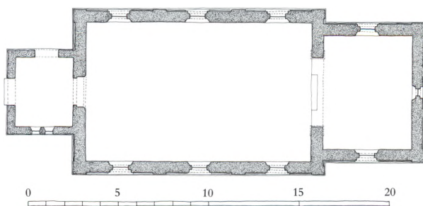
Fig. 3. Grundplan 1:300 tegnet af KdefL 1995 efter Svend Aage Aakjær 1982. – Grundriss.
