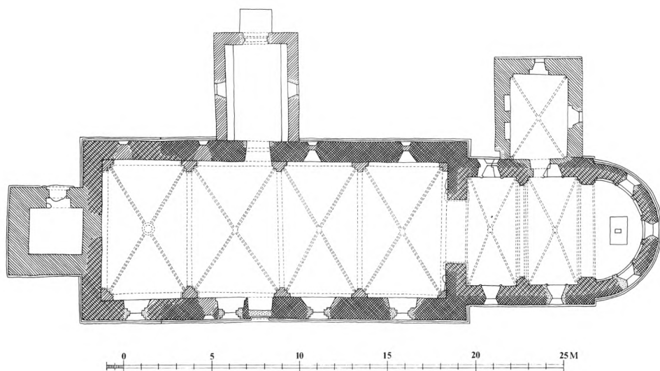
Fig. 10. Grundplan 1:300 af Brøndum kirke med korrigerende skravering, der angiver vestforlængelse og »modernisering« af korparti (s. 3537f.). Tegnet af Marianne Nielsen 2003 efter opmåling af Henrik Jacobsen 1979. – Grundriss 1:300 der Kirche zu Brøndum mit korrigierender Schraffierung, die eine Erweiterung nach Westen angeben sowie eine Modernisierung des Chores.
