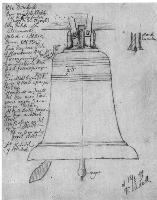
Fig. 3. Klokke, 1300'rne, i Ribe domkirkes Mariatårn (s. 3527). Opmåling ved F. Uldall 1899. — Glocke, 14. Jahrhundert. Im Marienurm des Domes zu Ribe.
