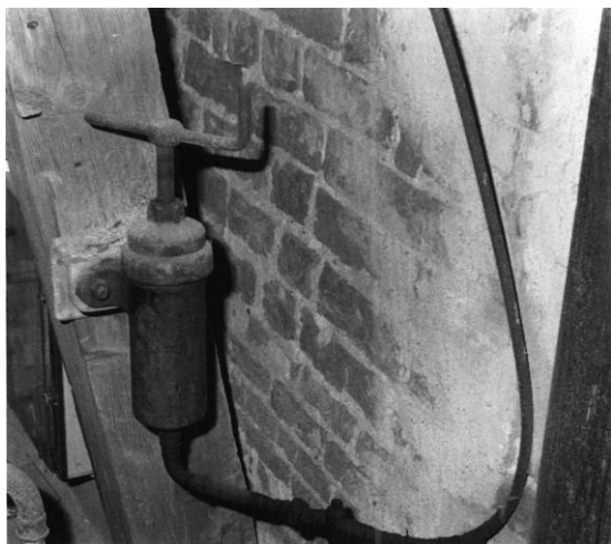
Fig. 15. Anordning til smøring af vindfløjen (s. 89), i tårnets nuværende klokkestokværk. Hans Stiesdal fot. 1997. - Vorrichtung zum Schmieren der Wetterfahne im heutigen Glockenstockwerk des Turms.
