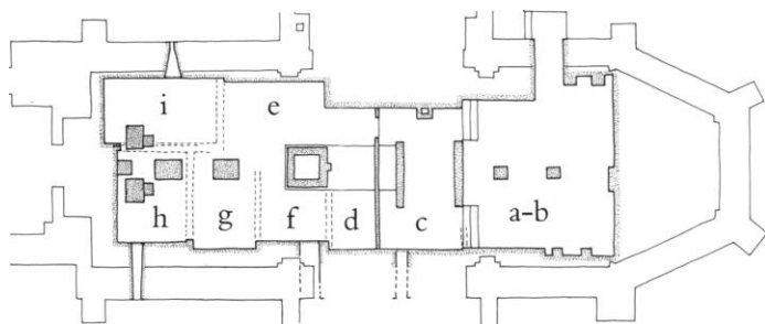
Fig. 16. Plan 1:300 af tømurede begravelser (s. 145) og fyrrummet (s. 88). Målt og tegnet af MV 1997, delvis på grundlag af opmåling ved Hother Paludan 1933. - Grundriß von Gräften und Heizkeller. Vermessen und gezeichnet 1997, teilweise auf Grundlage der Vermessungen von 1933.
