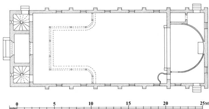
Fig. 7. Plan 1:300. Efter Carl Brummer 1905, tegnet af Marianne Nielsen 1998. Øst opad. - Grundriß 1905.
