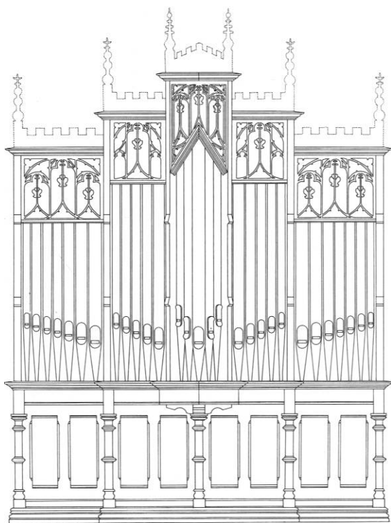
Fig. 12. *Orgel, 1888, bygget af A. H. Busch & Sønner til Industri- Landbrugs- og Kunstudstillingen i København. Siden 1949 i Vestre kirkegårds kapel (s. 484). Opmåling affacade, ved Peter Duun Andersen 1999. - *Orgel, 1888, gebaut von A. H. Busch & Sønner für die Industrie-Landwirtschafts- und Kunstausstellung in Kopenhagen. Seit 1949 in der Kapelle des Westfriedhofes.
