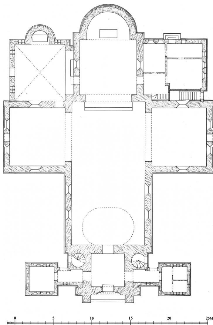
Fig. 2. Plan 1:300. Opmåling ved arkitektfirmaet Søren Jensen 1995, suppleret af NJP og tegnet af MN 1999. - Grundriss.
