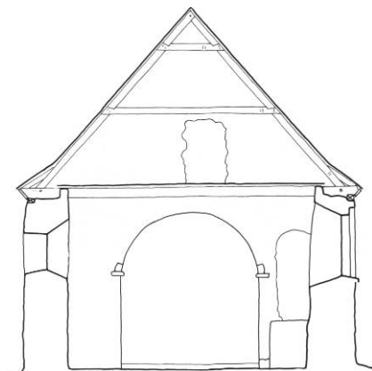
Fig. 4. Tværsnit 1:150 gennem skib set mod øst. Målt af Peter Duun Andersen 1998 og tegnet af MN 1999. - Querschnitt 1:150 durch das Schiff gegen Osten.
