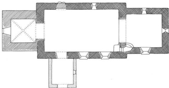
Fig. 5. Plan 1:300. Målt af arkitektfirmaet Søren Jensen 1997, suppleret af NJP og tegnet af MN 1999. - Grundriss.
