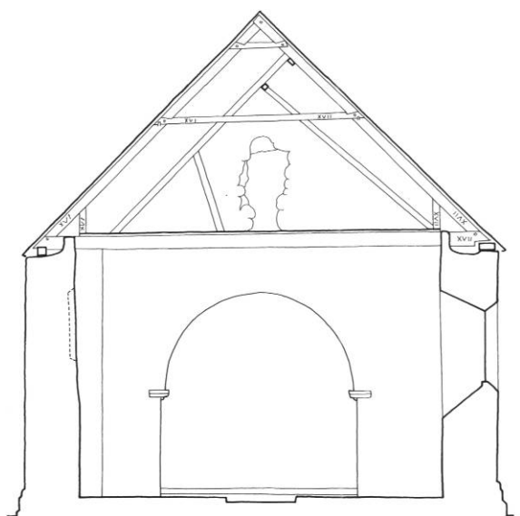
Fig. 7. Tværsnit 1:150 gennem skibet set mod øst. Målt af Peter Duun Andersen 1997 og tegnet af MN 2000. — Querschnitt durch Schiff gegen Osten.
