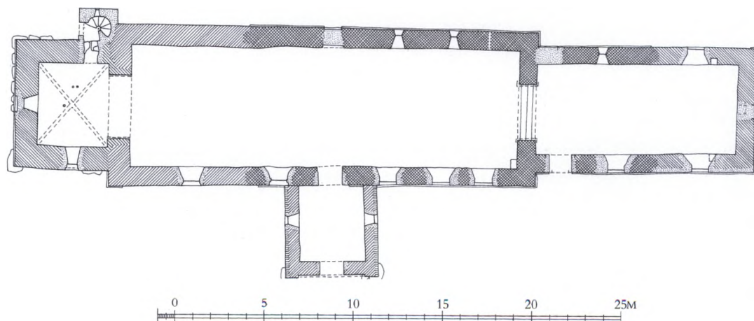
Fig. 8. Plan 1:300. Målt af John Bennetzen 1996, suppleret og tegnet af Thomas Bertelsen 2007. - Grundriß.
