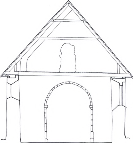
Fig. 15. Tværsnit 1:150 gennem skibet, set mod øst. Målt af John Bennetzen 1996 og tegnet af Thomas Bertelsen 2007.— Querschnitt durch Schiff, gegen Osten.
