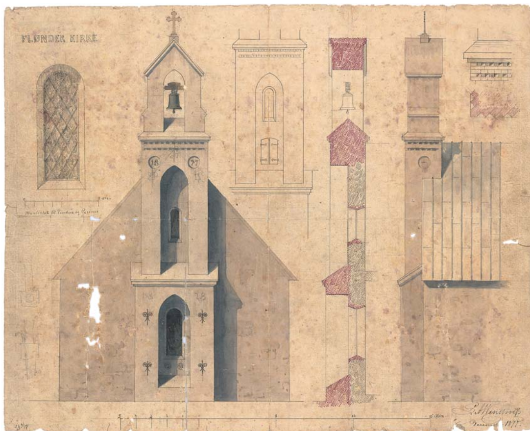
Fig. 13. Projekttegning til \dagger klokkekam ved skibets vestgavl (s. 890). 1:150. I midten alternativ udformning af øverste niche med foreslået adgang til skibets loft. Tegnet af L. A. Winstrup 1877. – Projektzeichnung für \dagger Glockenkamm an der westlichen Giebelwand des Schiffes. In der Mitte alternative Ausformung der obersten Nische mit Vorschlag für Zugang zur Decke des Schiffes.
