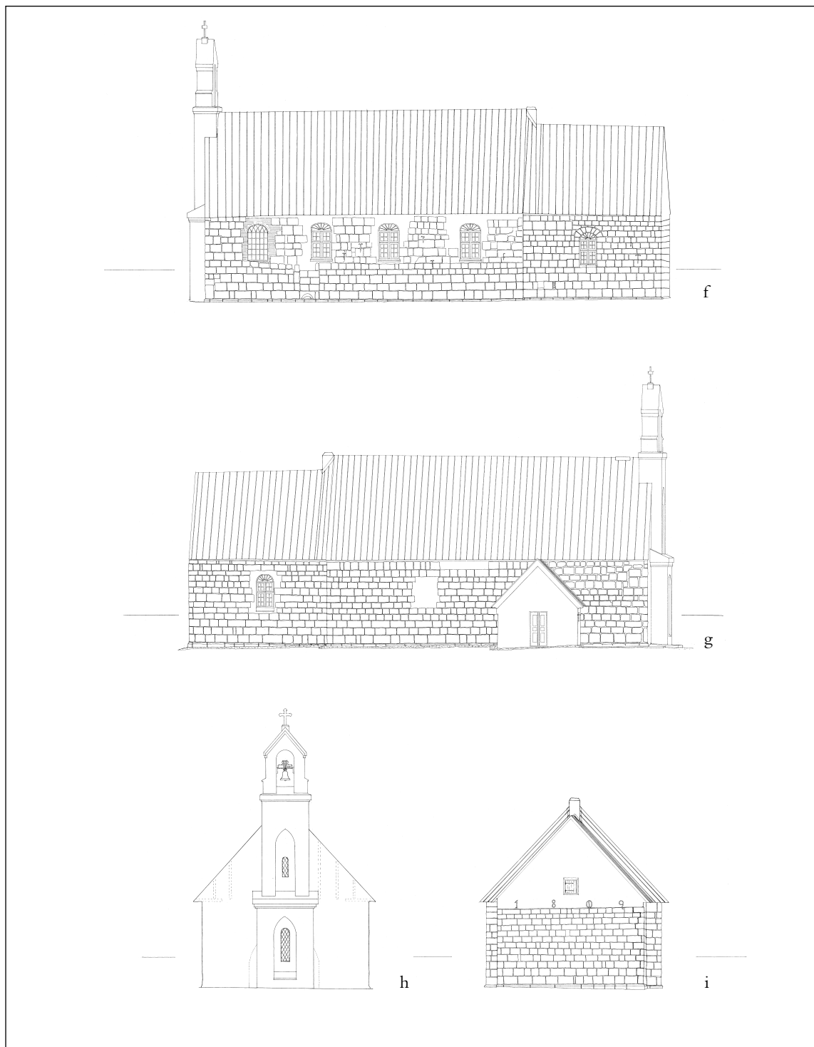
Fig. 8f-i. Opmålinger før restaureringen 1940-42, 1:300. f. Opstalt af sydfacaden. g. Opstalt af nordfacaden. h. Opstalt af vestfacaden. i. Opstalt af østfacaden. Målt og tegnet af M. B. Fritz & Søn 1937. — Vermessungen vor der Restaurierung 1940-42. f. Aufriss der Südfassade. g. Aufriss der Nordfassade. h. Aufriss der Westfassade. i. Aufriss der Ostfassade.
