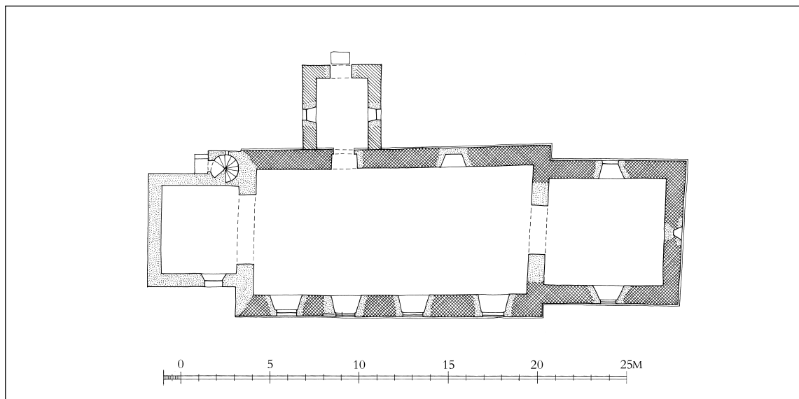
Fig. 4. Grundplan. 1:300. Målt af M. B. Fritz & Søn 1937–40, suppleret af Peter Duun og tegnet af Thomas Bertelsen 2009. – Grundriss .
