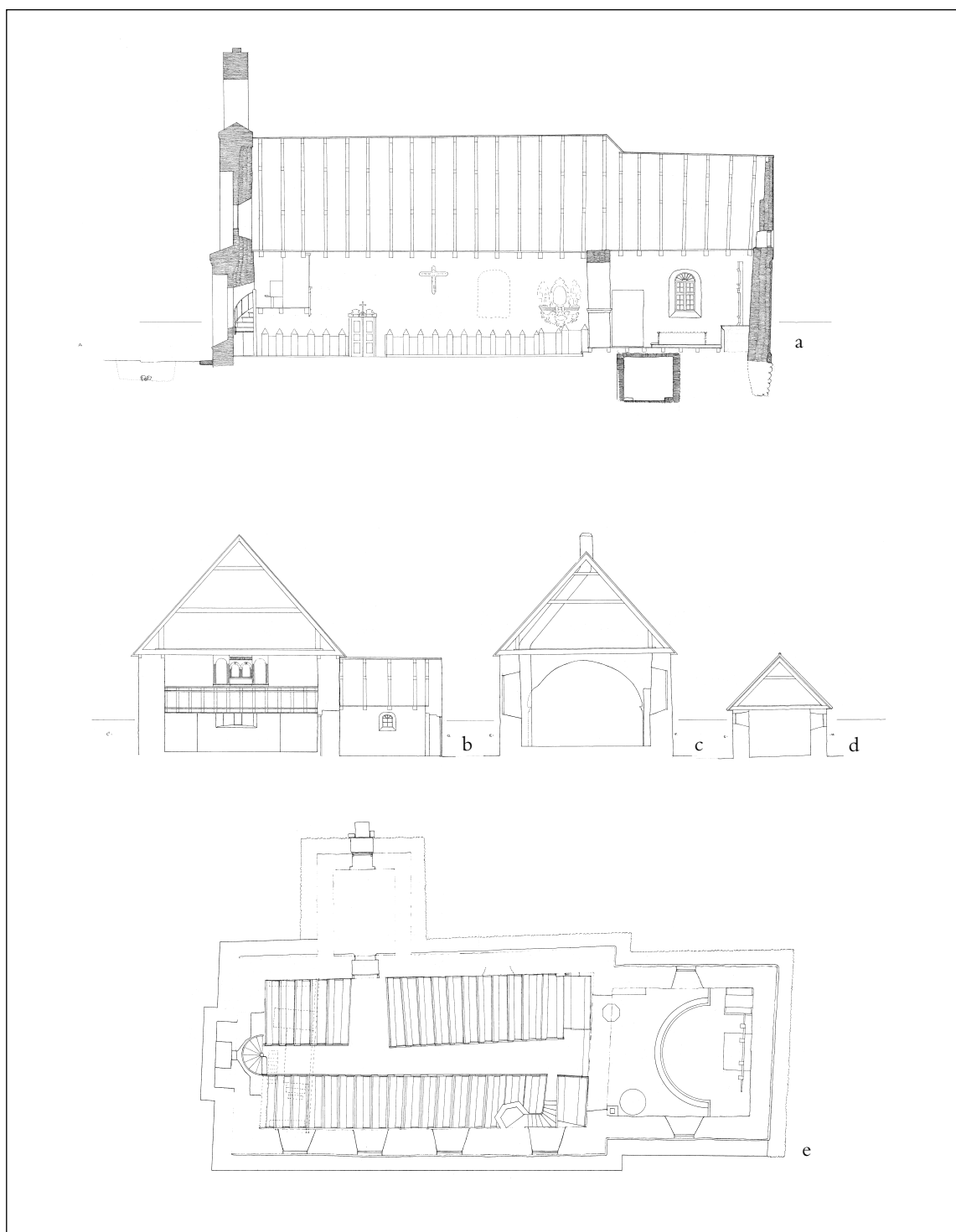
Fig. 8a-e. Opmålinger for restaureringen 1940-42, 1:300. a. Længdesnit set mod nord. b. Snit af skib og våbenhus set mod vest. c. Tværsnit af koret set mod vest. d. Tværsnit af våbenhuset. e. Plan. Målt og tegnet af M. B. Fritz & Søn 1937. – Vermessungen vor der Restaurierung 1940-42. a. Längsschnitt gegen Norden. b. Schnitt des Schiffes und Vårhauses gegen Westen. c. Querschnitt des Chores gegen Westen d. Querschnitt des Vårhauses. e. Grundriss.
