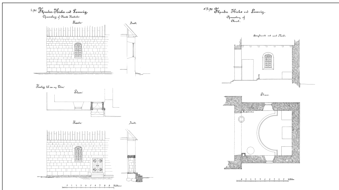
Fig. 12. Opmåling af koret, plan, snit og opstalter 1:300, med udkast til projekteret dør på nordsiden (s. 891). Målt og tegnet af Frits Uldall 1901. – Vermessung des Chores, Grundriss, Schnitt und Aufrisse, mit Entwurf für projektierte Tür an der Nordseite.
