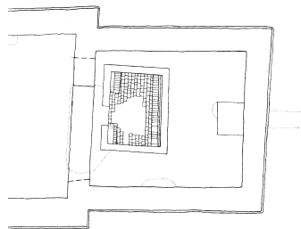
Fig. 54. Opmåling af koret med tømuret begravelse (s. 922). 1:300. Målt og tegnet af M. B. Fritz & Søn 1937. – Vermessung des Chors mit tømuretem Begräbnis.
