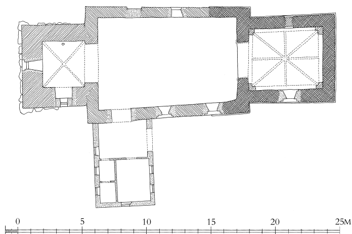
Fig. 6. Plan 1:300. Målt af Sven Fritz 1943, suppleret af Vilhelmsen, Marxen og Bech-Jensen 2002 samt suppleret og tegnet af Hugo Johannsen 2010. – Grundriss.
