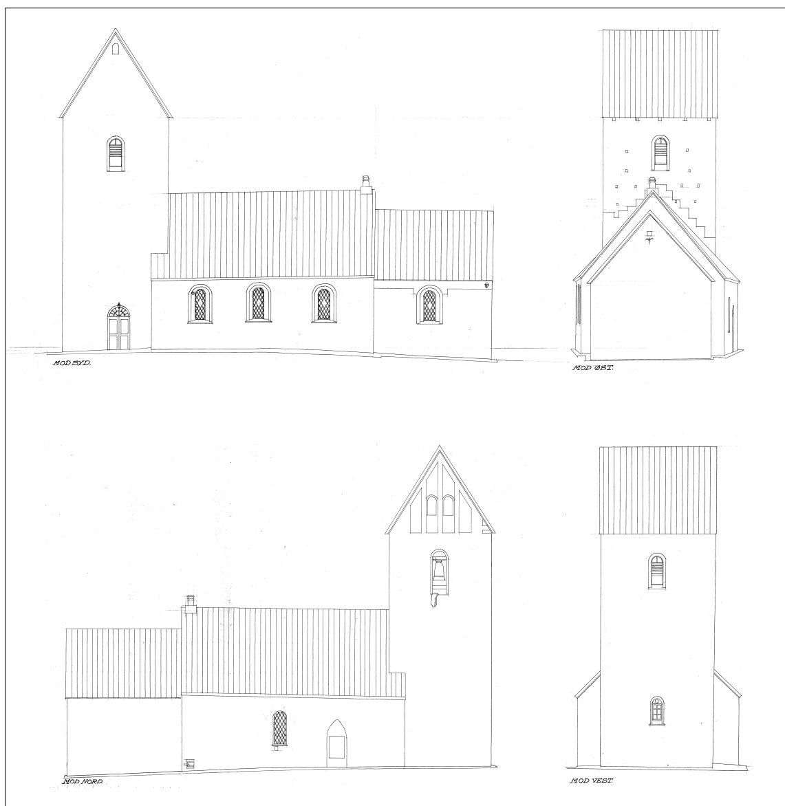
Fig. 8a-b. Facader, snit og plan. 1:300. Viggo Norn 1952. Horsens Museum. – Fassaden, Schnitte und Plan.
