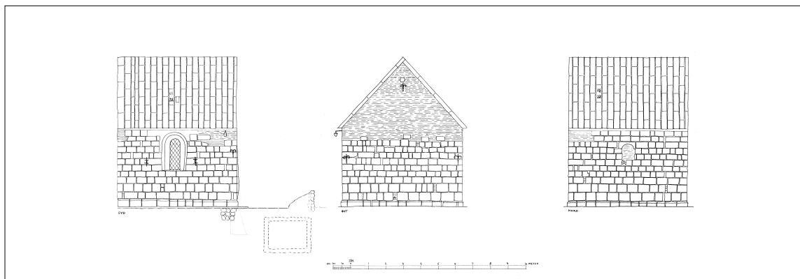
Fig. 12. Korets facader. 1:300. Målt og tegnet af Sven Fritz 1943. – Fassade des Chores.
