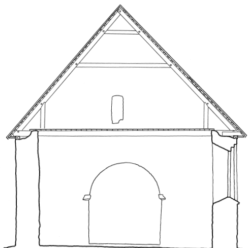
Fig. 5. Tværsnit 1:150 gennem skibet set mod øst. Målt og tegnet af Peter Duun 1999 og 2010. – Querschnitt 1:150 durch Schiff und Kreuzarm gegen Ost.
