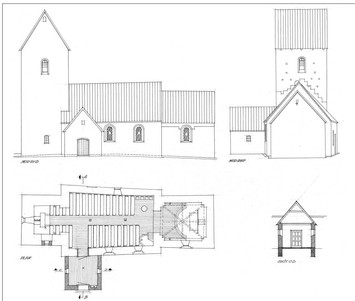
Fig. 11. Plan, facader og snit med forslag til våbenhus. 1:300. Viggo Norn 1952. Horsens Museum. – Grundriss, Fassaden und Schnitt mit Vorschlag zu Vörhalle.
