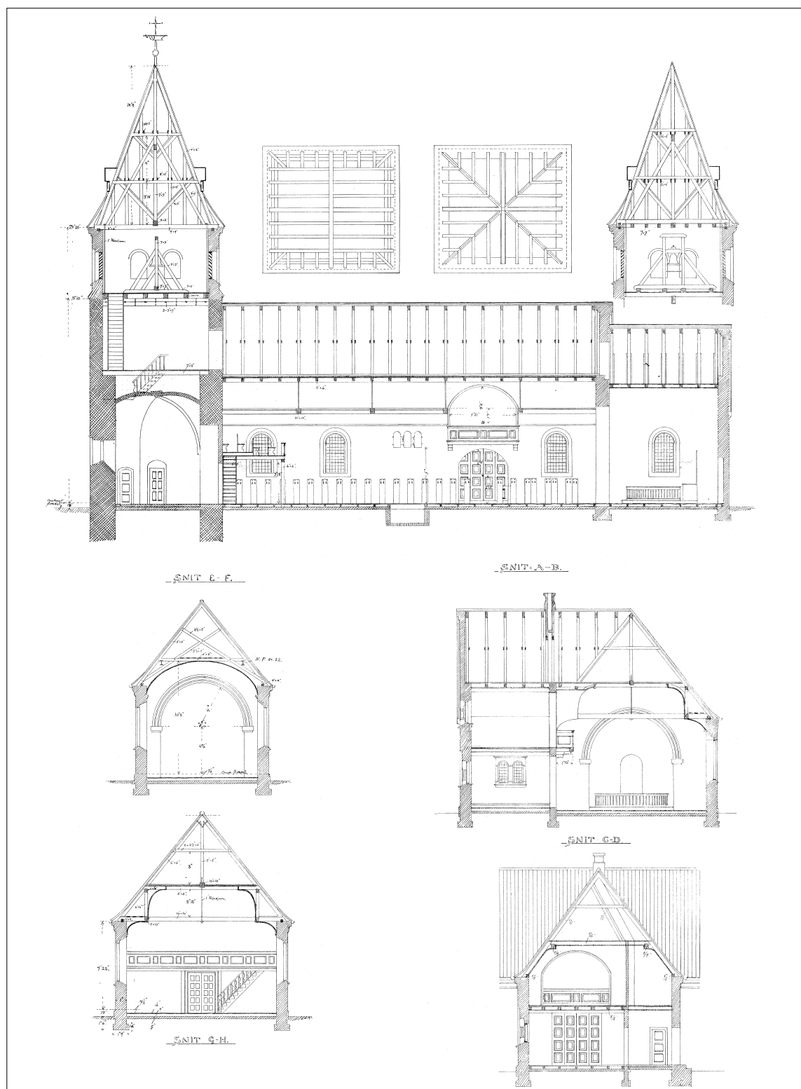
Fig. 7c. Længde- og tværsnit. 1:300. Ved K. Varming, 1909. Thyborøn-Harboøre Lokalarkiv. – Längs- und Querschnitte.
