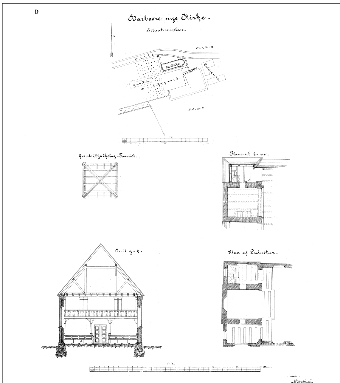
Fig. 6d. Situationsplan, planer og tværsnit til projekteret kirke ved A. E. Andersen 1907. 1:300. Thyborøn-Harboøre Lokalkiv. – Situationsplan, Pläne und Querschnitt für projektierte Kirche.
