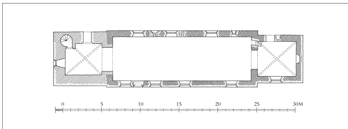
Fig. 12. Plan 1:300, målt af K. Varming 1908, jf. fig. 13, suppleret af Hugo Johannsen efter Chr. Axel Jensen 1909 og tegnet af Merete Rude 2011. – Grundriss .
