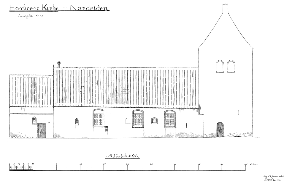
Fig. 14. Nordfacade 1:300, målt af Chr. Axel Jensen 1909 og tegnet af S.A. Claudt-Hansen. – Nordfassade.
