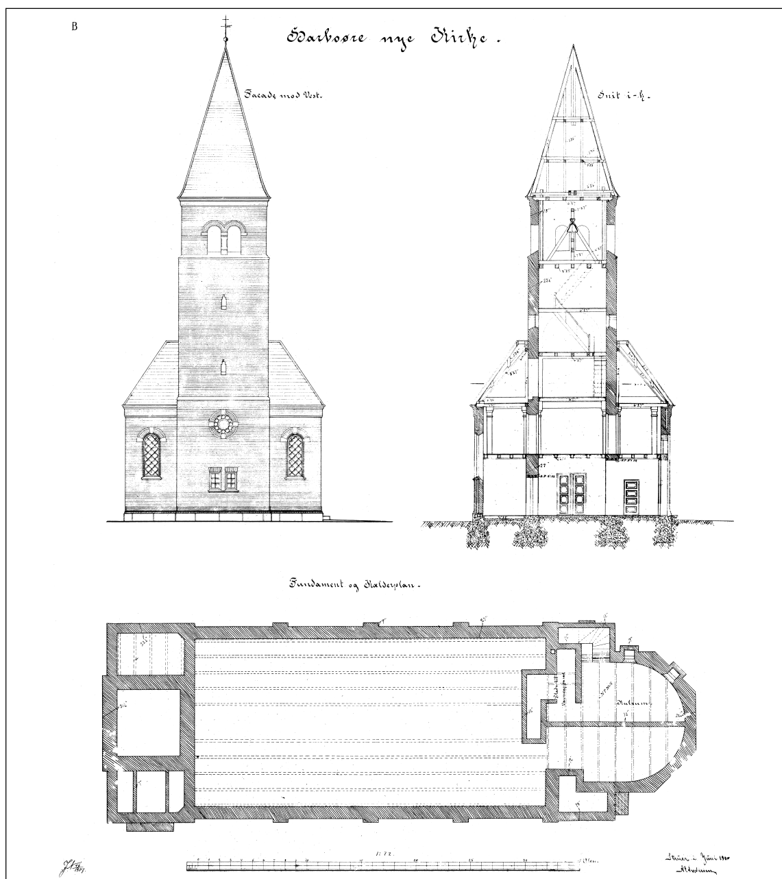
Fig. 6b. Kælderplan, vestfacade og tværsnit til projekteret kirke ved A. E. Andersen 1907. 1:300. Thyborøn-Harboøre Lokalkiv. – Untergeschoss, Westfassade und Querschnitt für projektierte Kirche.
