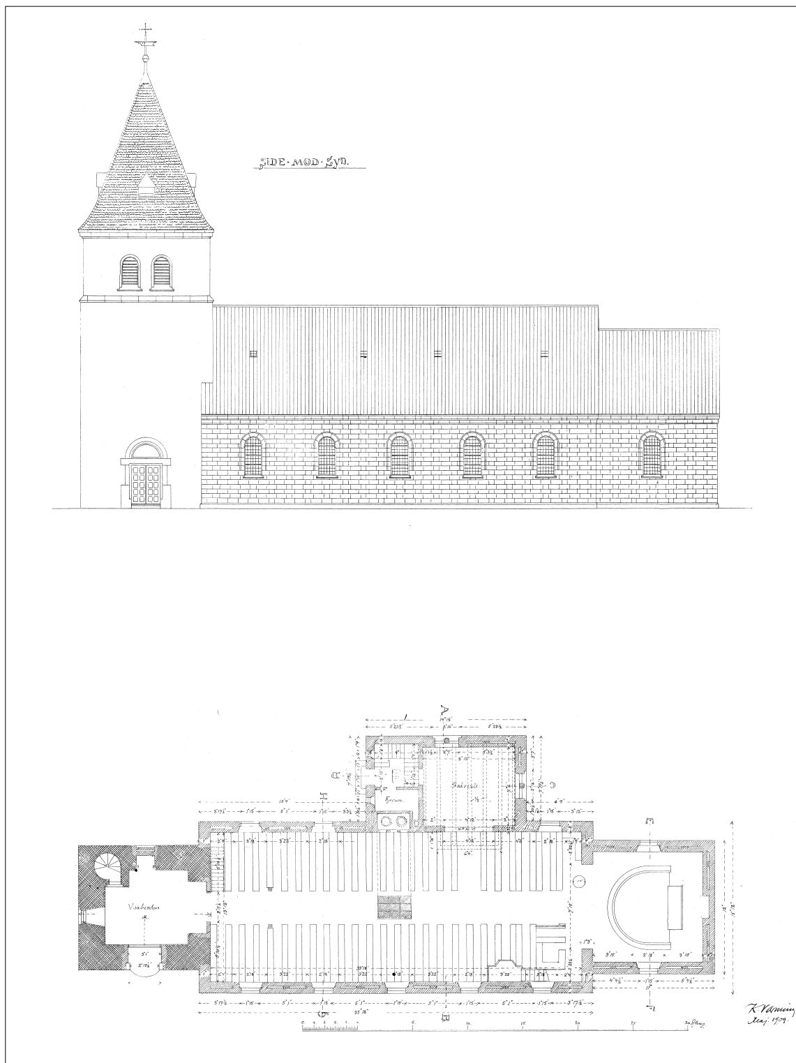
Fig. 7a. Sydfacade og plan. 1:300. Ved K. Varming, 1909. Thyborøn-Harboøre Lokalkiv. – Südfassade und Grundriss.
