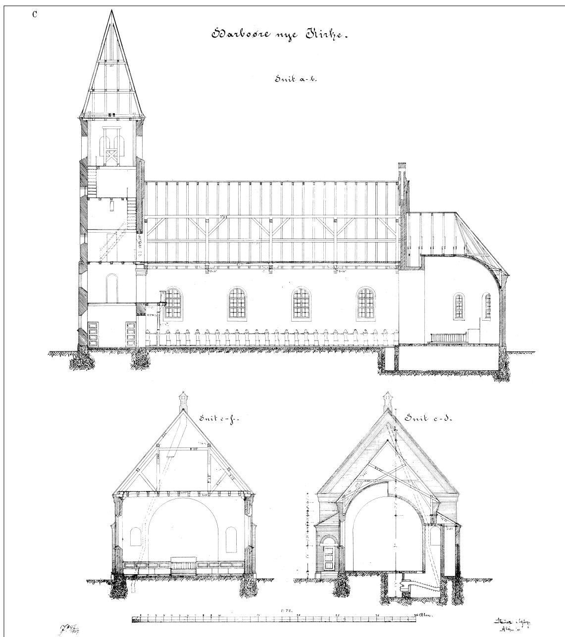
Fig. 6c. Længde- og tværsnit til projekteret kirke ved A. E. Andersen 1907. 1:300. Thyborøn-Harboøre Lokalkiv. – Längs- und Querschnitte für projektierte Kirche.
