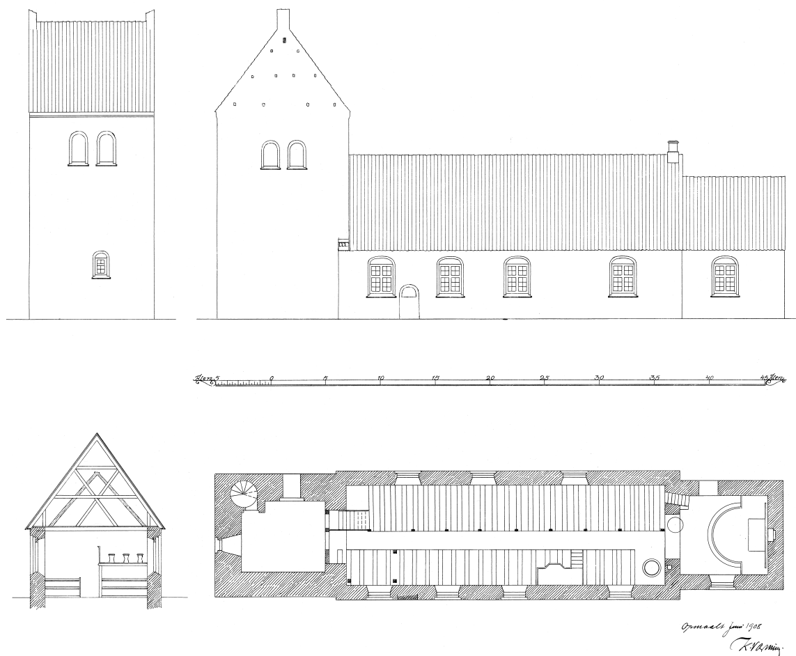
Fig. 13. Plan, facader og snit. 1:300. Målt af K. Varming 1908. – Grundriss, Fassaden und Schnitt.
