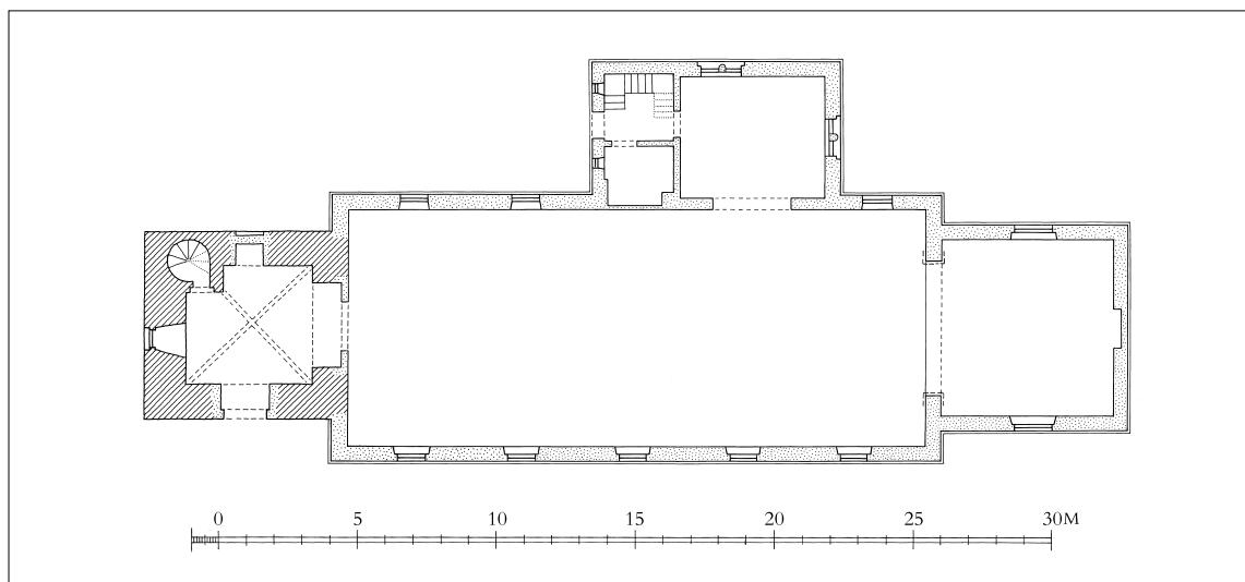
Fig. 8. Plan 1:300. Målt af Poul Hansen og Ib Lydholm 1974, suppleret af Hugo Johannsen og tegnet af Merete Rude 2010. – Grundriss .
