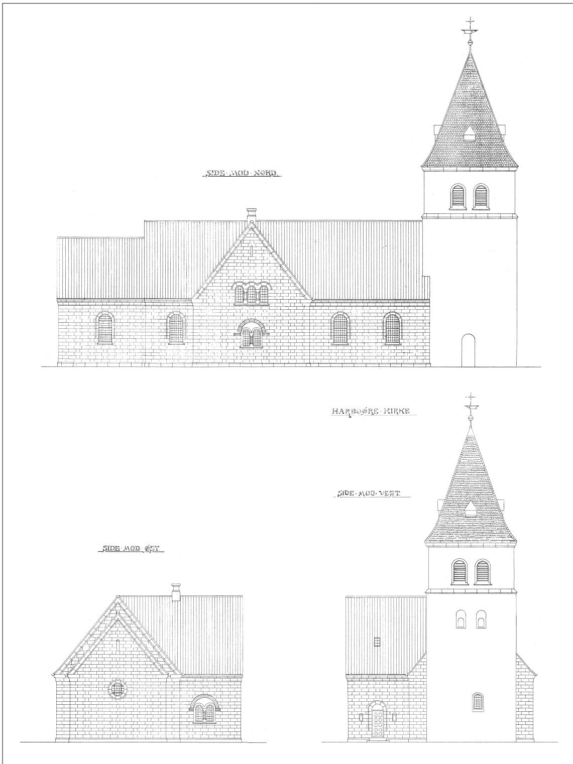
Fig. 7b. Nord-, øst- og vestfacade. 1:300. Ved K. Varming, 1909. Thyborøn-Harboøre Lokalkiv. – Nord-, Ost- und Westfassade.
