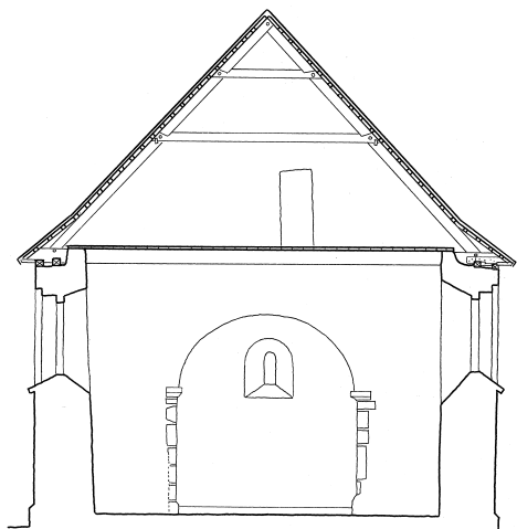
Fig. 4. Tværsnit 1:150, gennem skib set mod øst. Målt og tegnet af Peter Duun 2009. – Querschnitt durch das Schiff gegen Osten.
