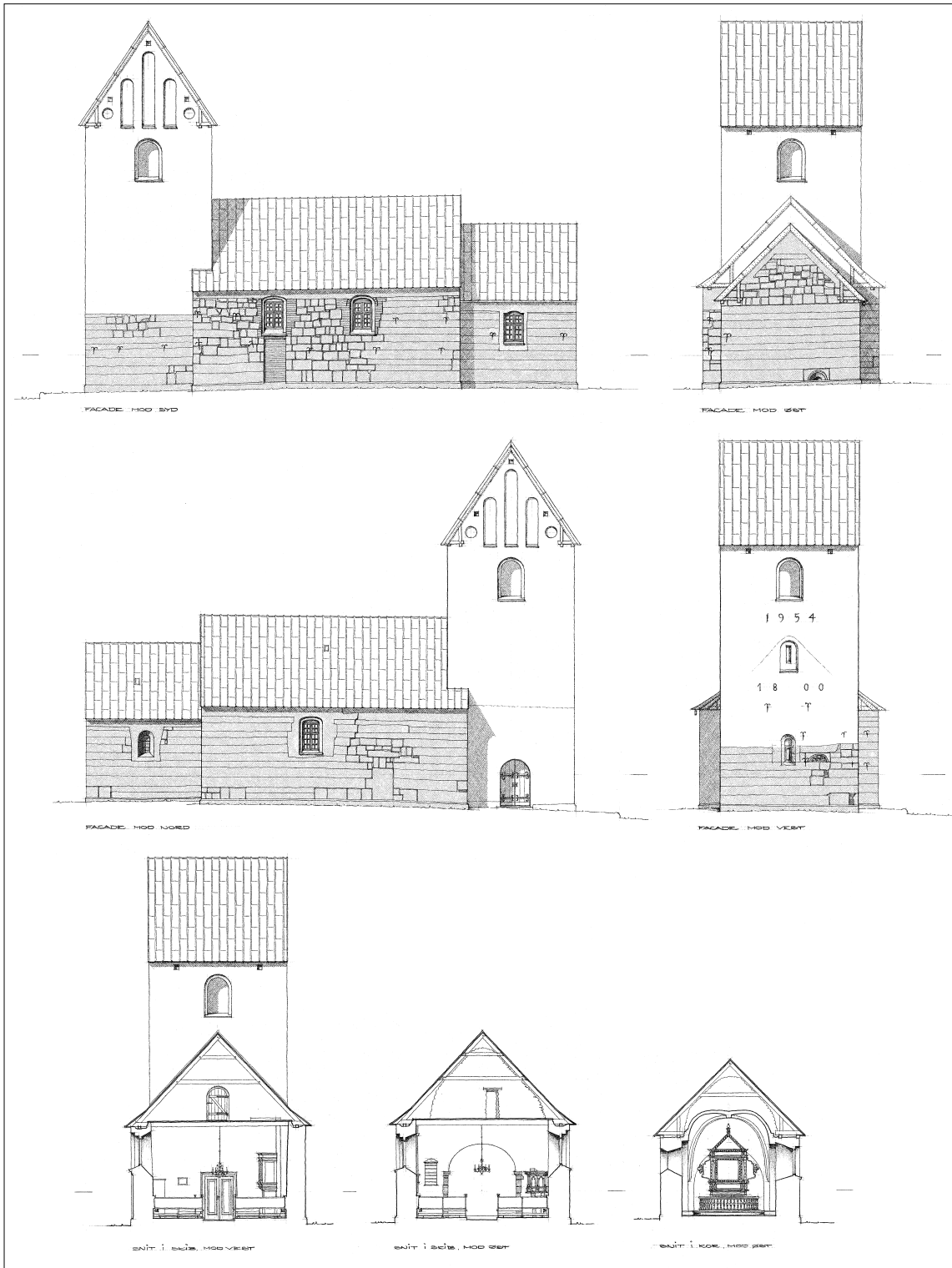
Fig. 6. Facader samt tværsnit gennem skib og kor. 1:300. Målt og tegnet af Poul Hansen og Ib Lydholm 1979. Poulsen & Partnere, Thisted. – Fassaden und Schnitt durch Schiff und Chor.
