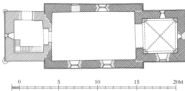
Fig. 5. Plan 1:300. Målt af Poul Hansen og Ib Lydholm 1979, suppleret af Hugo Johannsen 2010 og tegnet af Merete Rude 2010. – Grundriss.
