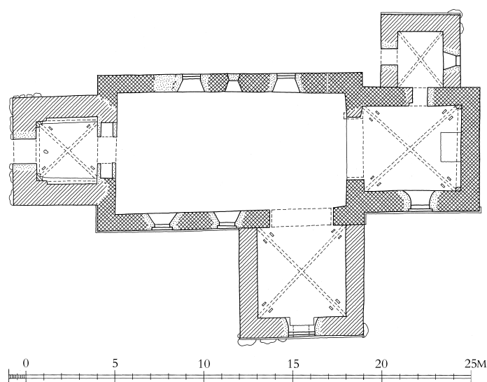
Fig. 6. Plan 1:300. Målt af Peter Duun 2009, suppleret af Hugo Johannsen 2010 og tegnet af Merete Rude 2010. – Grundriss .
