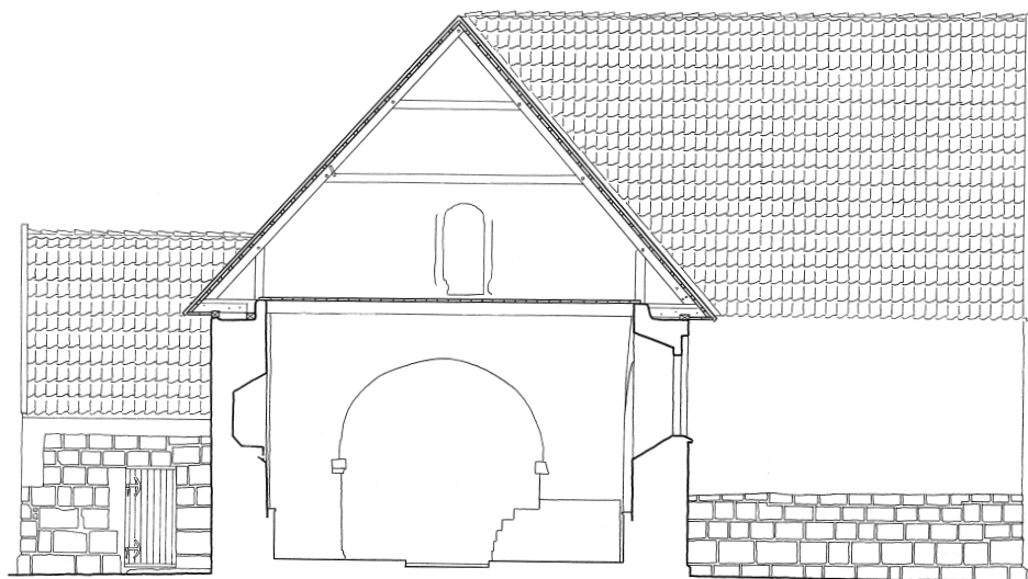
Fig. 5. Tværsnit 1:150. Målt og tegnet af Peter Duun 2009. – Querschnitt .
