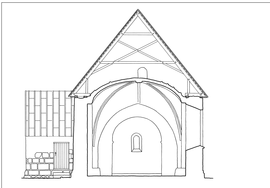
Fig. 4. Tværsnit 1:150 gennem skibet set mod øst. Målt og tegnet af Peter Duun 2010. – Schnitt durch Schiff gegen Osten.
