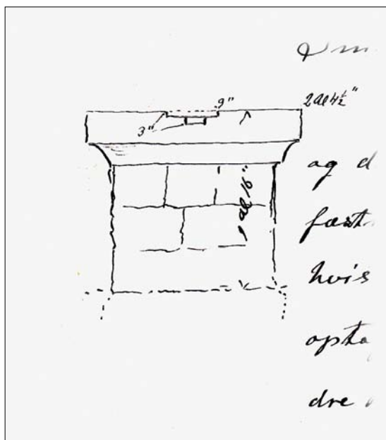
Fig. 17. Opstalt af det middelalderlige alterbord med snit af bordpladen, hvori ses helgengrav (s. 1462). Tegning 1907 af J. Magnus-Petersen. – Aufriss des mittelalterlichen Altartisches mit Schnitt der Tischplatte, darin das Heiligengrab.
