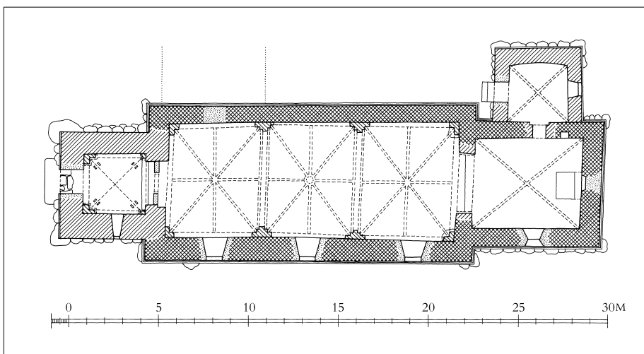
Fig. 5. Plan 1:300. Målt af Poul Hansen og Ib Lydholm 1977, suppleret af Hugo Johannsen 2011 og tegnet af Merete Rude 2012. – Grundriss.
