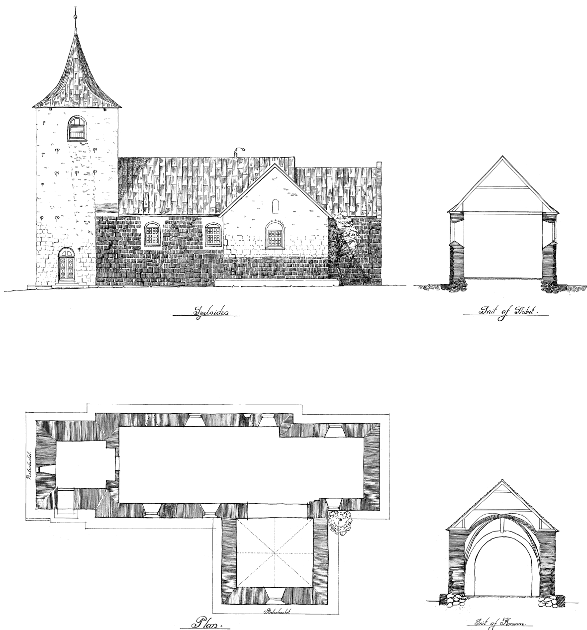
Fig. 7a. Plan, snit og facade. 1:300. Målt og tegnet af Søren Vig Nielsen 1929. LAVib. – Grundriss, Schnitt und Fassade .
