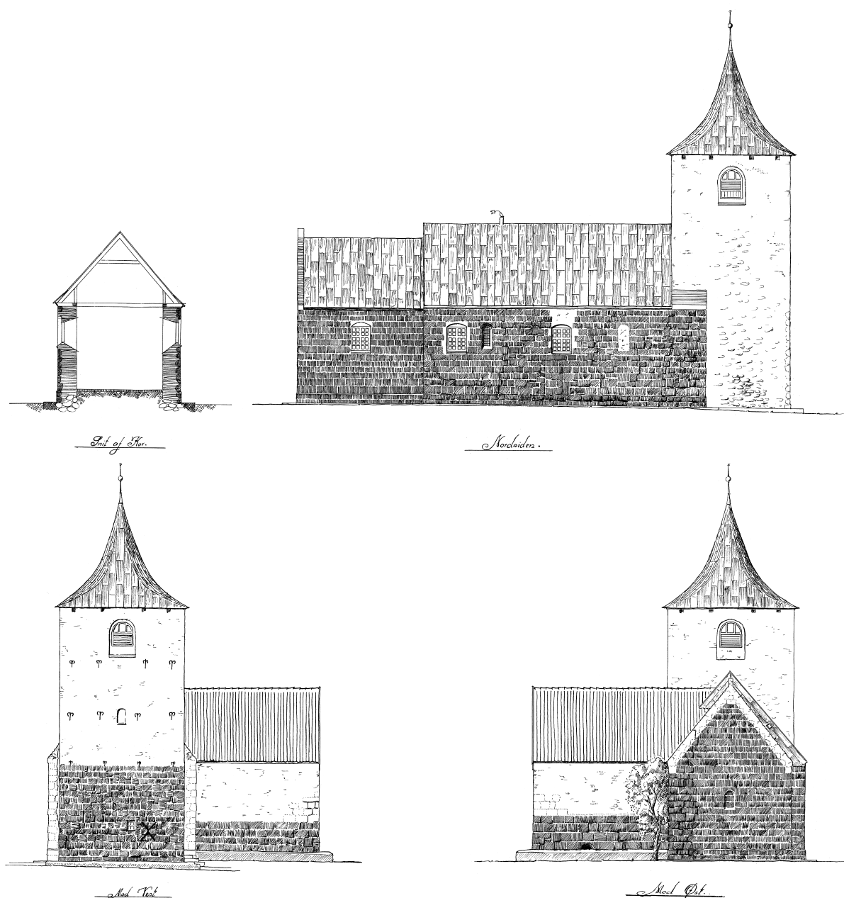
Fig. 7b. Snit og facader. 1:300. Målt og tegnet af Søren Vig Nielsen 1929. LAVib. – Schnitt und Fassaden.
