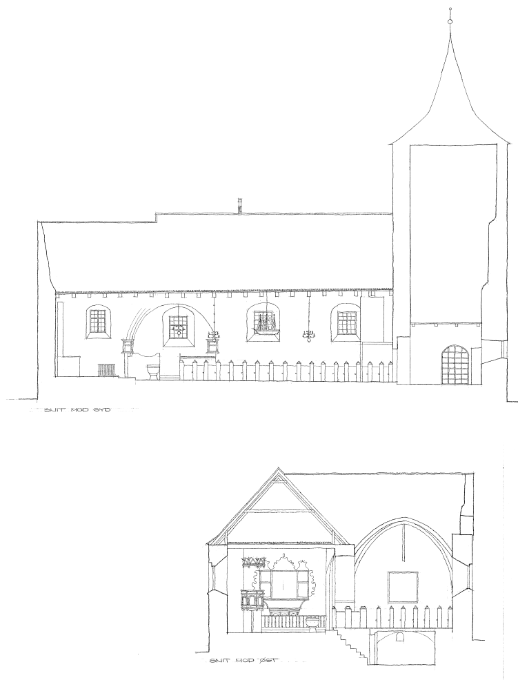
Fig. 15. Længdesnit mod syd og tværsnit mod øst 1:300. Målt og tegnet af Poul Hansen og Ib Lydholm 1976. Poulsen og Partnere, Thisted. – Längsschnitt gegen Süden und Querschnitt gegen Osten.
