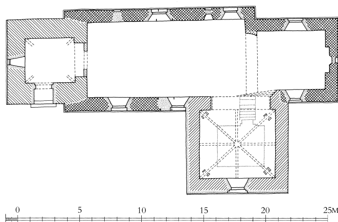
Fig. 6. Plan 1:300. Målt af Peter Duun 2009, suppleret af Anders C. Christensen og Hugo Johannsen samt tegnet af Merete Rude 2012. – Grundriss.
