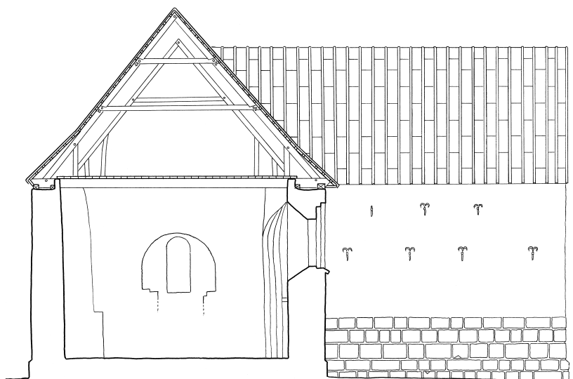
Fig. 5. Tværsnit 1:150 gennem skibet set mod øst. Målt og tegnet af Peter Duun 2009. – Querschnitt 1:150 durch das Schiff gegen Osten.
