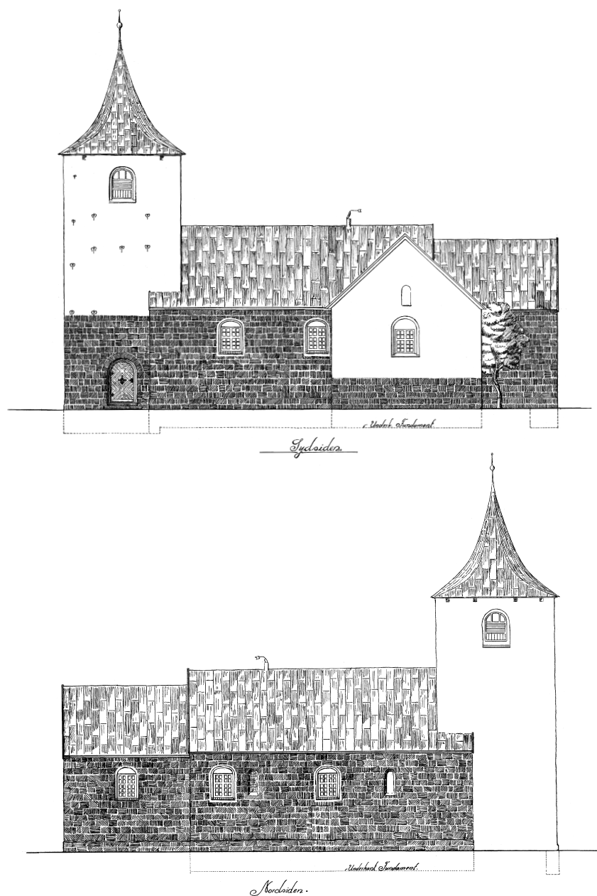
Fig. 14. Restaureringsforslag 1929. Facader. 1:300. Målt og tegnet af Søren Vig Nielsen 1929. LAVib. – Vorschlag zur Restaurierung 1929. Fassade.
