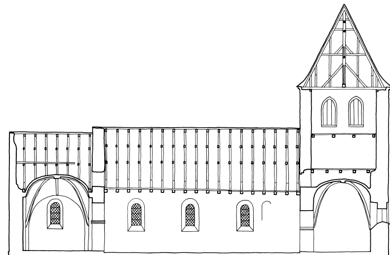
Fig. 7. Længdesnit set mod syd. 1:300. Målt af Poul Hansen og Ib Lydholm 1967, suppleret og tegnet af Anders C. Christensen 2013. – Schnitt gegen Süden.
