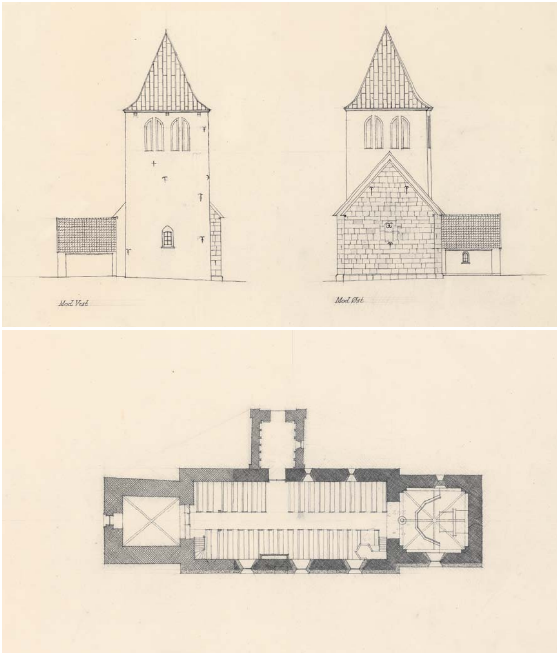
Fig. 10c-e. Øst- og vestfacader samt plan. 1:300. Målt og tegnet af Holger Sørensen 1935. Danmarks Kunstbibliotek. – Fassaden und Plan.
