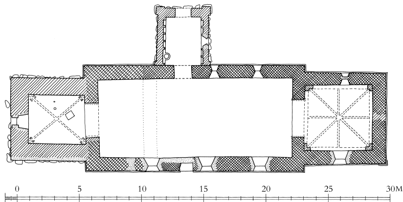
Fig. 6. Plan. 1:300. Målt af Poul Hansen og Ib Lydholm 1967, suppleret og tegnet af Anders C. Christensen 2013. – Plan.
