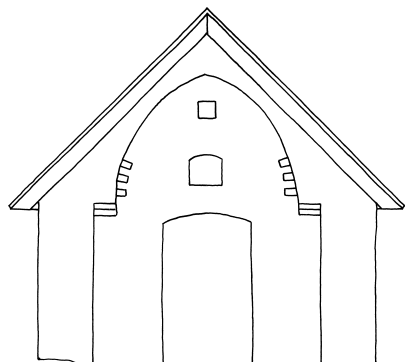
Fig. 47. Våbenhusets nordgavl (s. 1741). 1:100. Målt af Søren Andersen Arkitekt 2003, suppleret og tegnet af Anders C. Christensen 2013. – Nordgiebel des Vorhalles.
