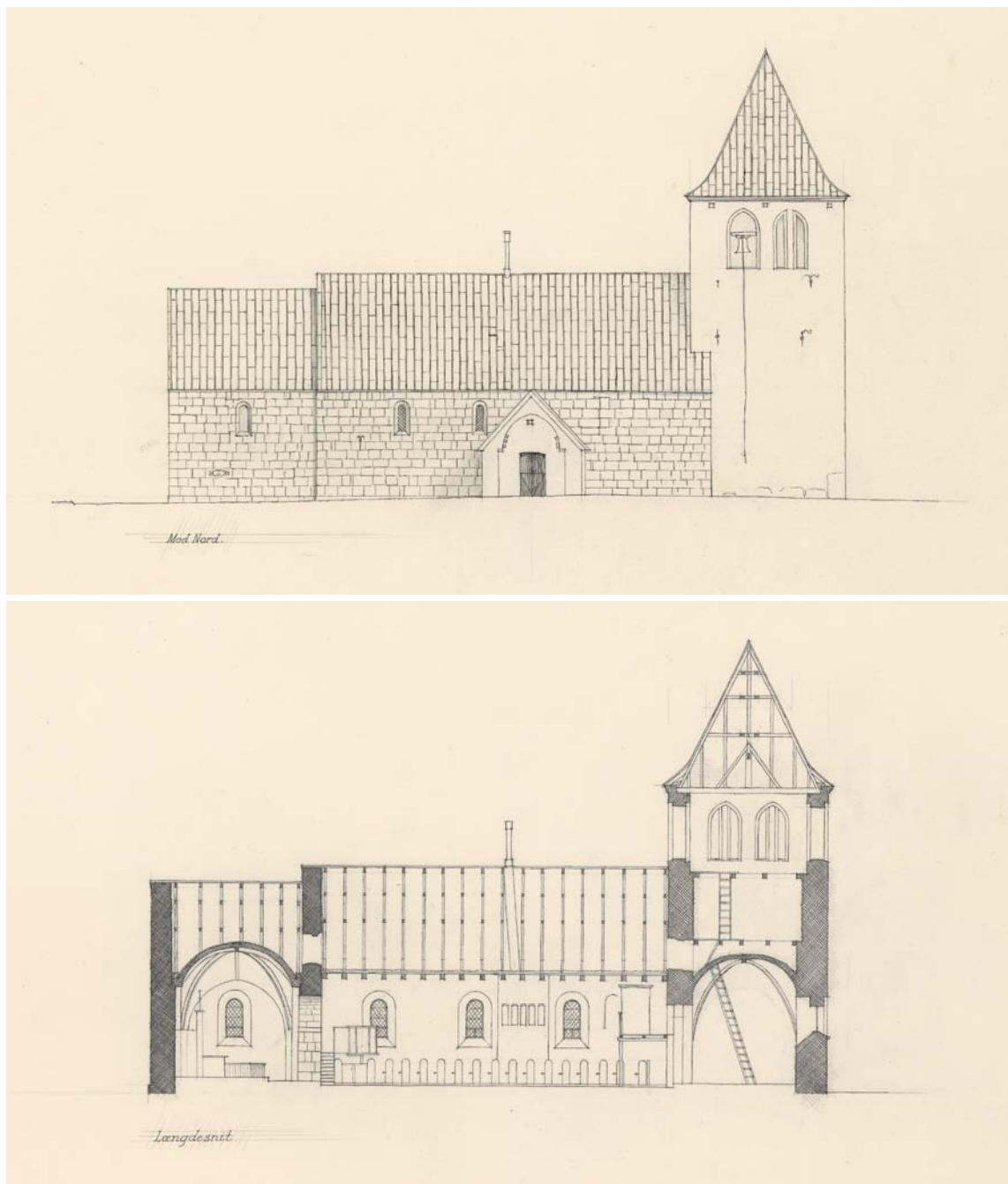
Fig. 10a-b. Nordfacade og længdesnit. 1:300. Målt og tegnet af Holger Sørensen 1935. Danmarks Kunstbibliotek. – Nordfassade und Plan.
