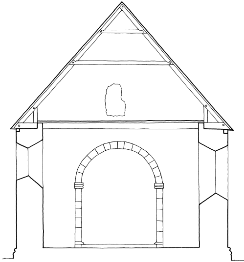
Fig. 5. Tværnsnit gennem skibet set mod øst. 1:150. Målt af Holger Sørensen 1935 (jf. fig. 10a-e), tegnet af Anders C. Christensen 2013. – Querschnitt durch das Schiff aus Osten.
