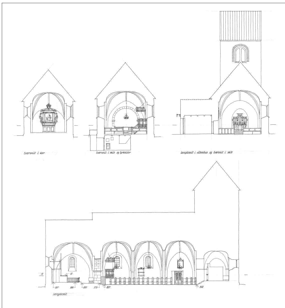
Fig. 13. Tvær- og længdesnit. 1:300. Målt og tegnet af Jens Foged og Poul Hansen 1955. – Quer- und Längsschnitt.
