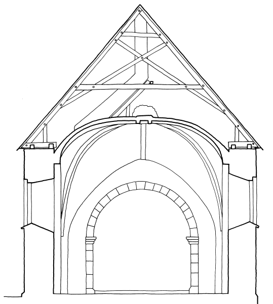
Fig. 8. Tværsnit. 1:150 gennem skibet set mod øst. Målt af Jens Foged og Poul Hansen 1955, suppleret og tegnet af Anders C. Christensen 2013. – Querschnitt durch das Schiff gegen Osten.
