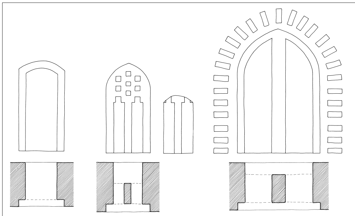
Fig. 15a-c. Plan og opstalter. 1:50. a. Dør mellem tårnets mellemstokværk og skibets loft. b. Nordre glug i tårnets mellemstokværk. c. Tårnets nordre glamhul (s. 1783). Målt og tegnet af Thomas Bertelsen 2005. – Grundriss und Aufriss. a. Tür zwischen Zwischenstockwerk des Turmes und Schiffsdecke. b. Nördliches Schalloch im Zwischenstockwerk des Turmes. c. Nördliches Hörloch des Turmes.
