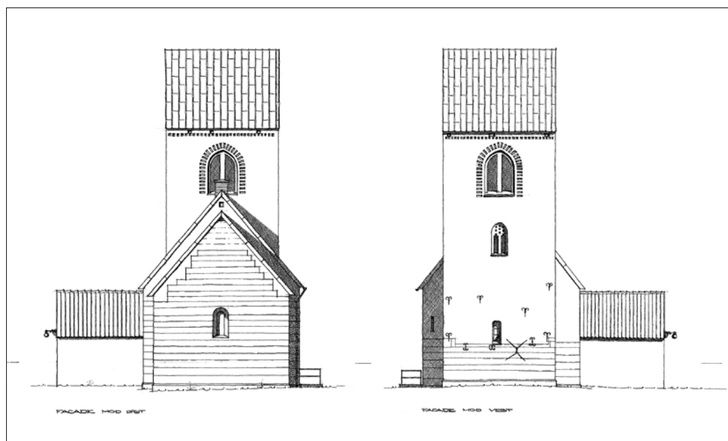
Fig. 12c-d. Facader. 1:300. Målt og tegnet af Poul Hansen og Ib Lydholm 1979-80. – Fassaden .
