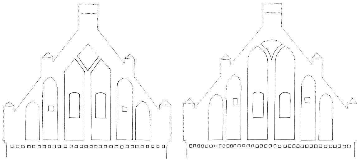
Fig. 62-63. Opstalter af tårnets gavltrekanter (s. 1788). 1:100. Ændringer efter ca. 1550 er udeladt. 62. Nord. 63. Syd. Målt og tegnet af Thomas Bertelsen 2005. – Aufriss der Giebeldreiecke des Turmes. Die Veränderungen nach ca. 1550 wurden ausgelassen. 62. Nord. 63. Süd.
