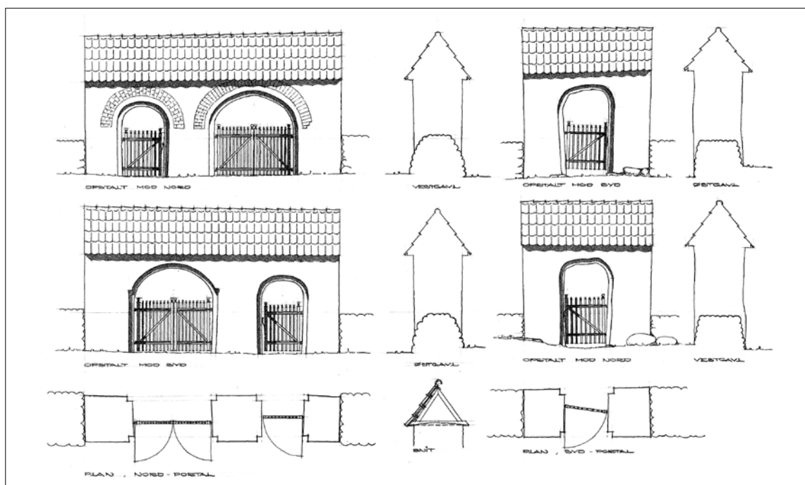
Fig. 60. Kirkegårdsportaler (s. 1775). 1:150. Målt af Poul Hansen og Ib Lydholm 1979. – Kirchhofsportale .
