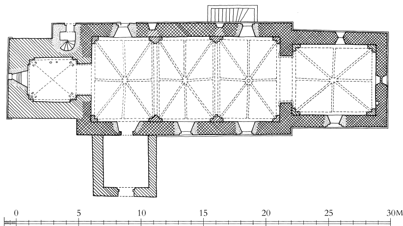
Fig. 9. Plan. 1:300. Målt af Jens Foged og Poul Hansen 1955, suppleret af Thomas Bertelsen 2005, suppleret og tegnet af Anders C. Christensen 2013. – Grundriss.
