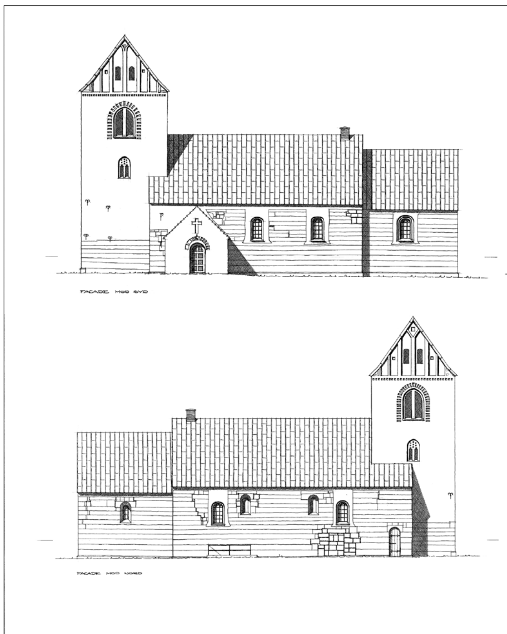
Fig. 12a-b. Facader. 1:300. Målt og tegnet af Poul Hansen og Ib Lydholm 1979-80. – Fassaden .
