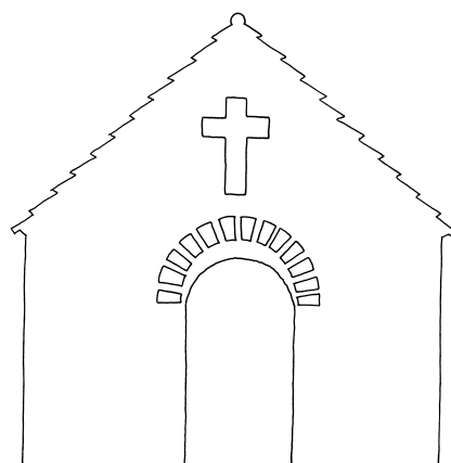
Fig. 61. Våbenhusets facade (s. 1788). 1:100. Målt af Poul Hansen og Ib Lydholm 1979–80, suppleret og tegnet af Anders C. Christensen 2013. – Die Fassade der Vörhalle .
