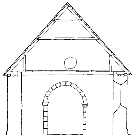
Fig. 5. Tværsnit gennem skibet set mod øst. 1:150. Målt og tegnet af Anders C. Christensen 2015. – Cross-section through the nave looking east.
