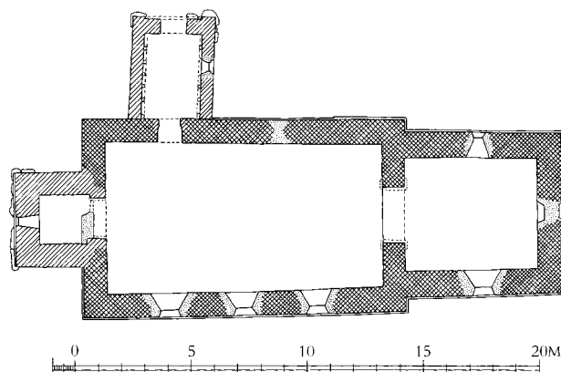
Fig. 6. Plan. 1:300. Målt af Emanuel Fleischer 1893, suppleret og tegnet af Anders C. Christensen 2015. – Plan.
