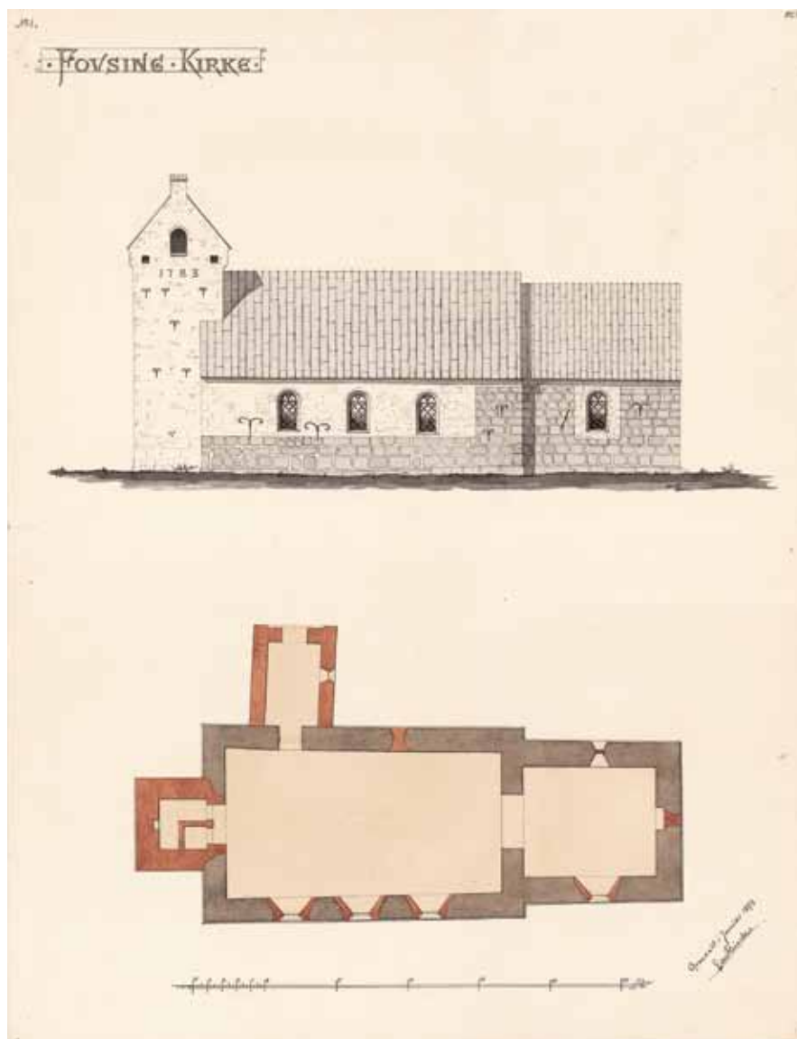
Fig. 7a-b. Plan og opstalt. 1:300. Målt og tegnet af Emanuel Fleischer 1893. – Plan and elevation.
