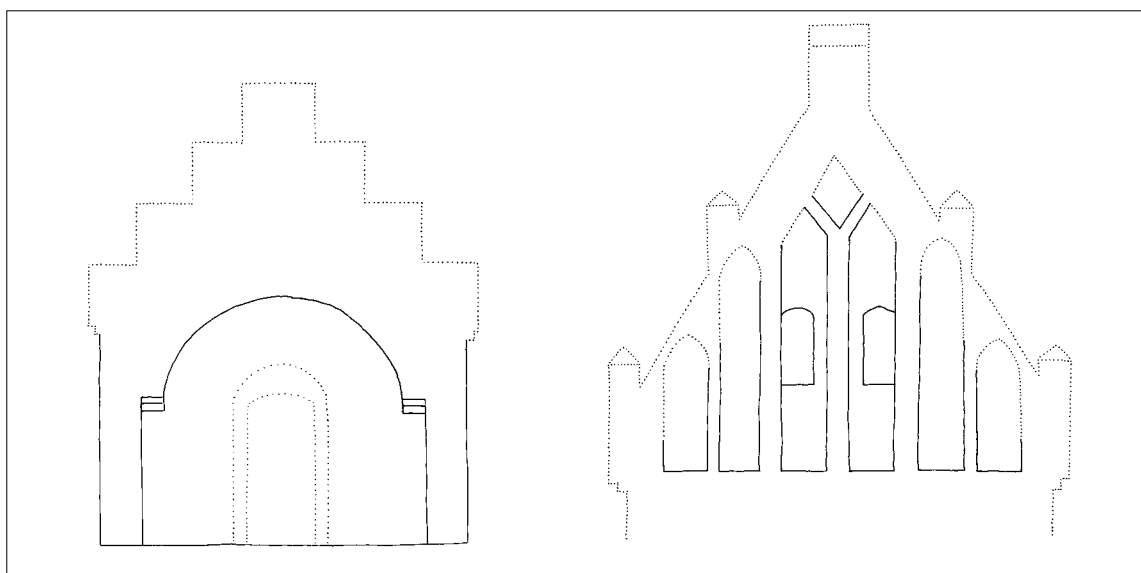
Fig. 50-51. Rekonstruktioner. 1:100. 50. Våbenhusets gavl (s. 2407). Målt og tegnet af Anders C. Christensen 2016. 51. Tårnets nordre gavltrekant (s. 2409). Målt af Thomas Bertelsen 2005, suppleret og tegnet af Anders C. Christensen 2016. – Reconstructions. 50. Gable of the porch. 51. Northern pediment of tower.
