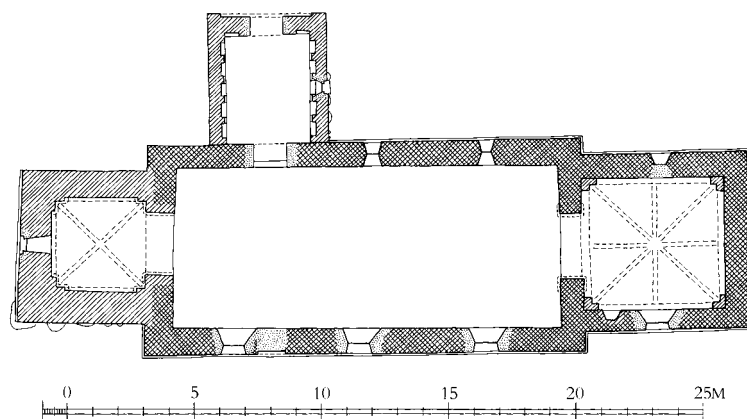
Fig. 6. Plan. 1:300. Målt af A. Havsteen-Mikkelsen 1983, suppleret og tegnet af Anders C. Christensen 2016. – Plan.
