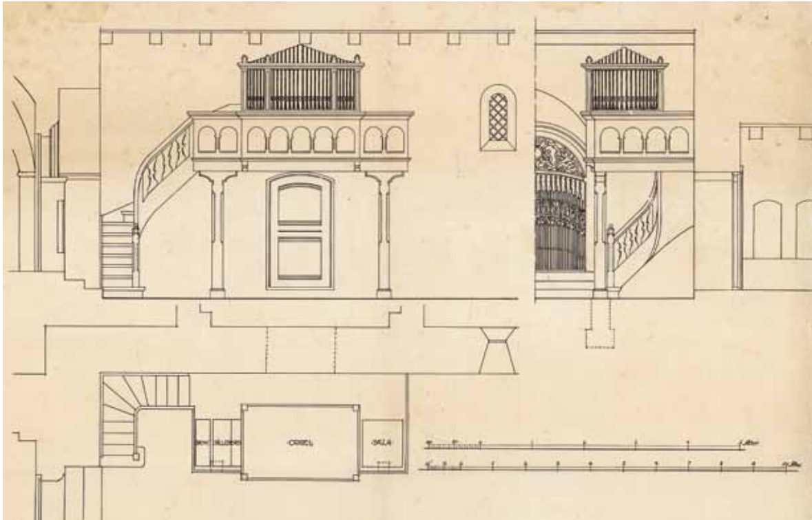
Fig. 38. Plan, snit og detaljer af \dagger orgelpulpitur og -facade (s. 2433). 1: 100. Tegning af Hans Arentoft 1917. I kirkens arkiv. – Plan, elevation and details of the \dagger organ gallery and facade. Drawing by Hans Arentoft, 1917.
