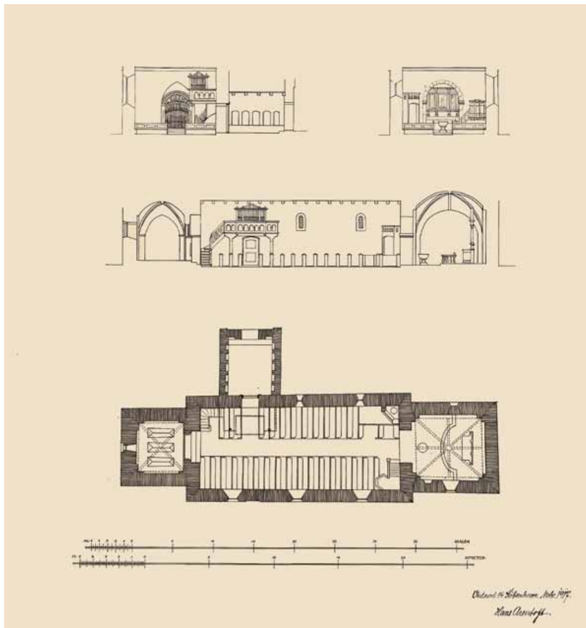
Fig. 10. Plan og snit. 1:300. Målt og tegnet af Hans Arentoft 1917. I kirkens arkiv. – Plan and sections.
