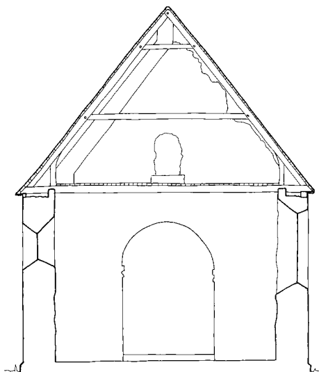
Fig. 5. Tværsnit af skibet set mod øst. 1:150. Målt og tegnet af Anders C. Christensen 2016. – Cross-section through nave looking east.
