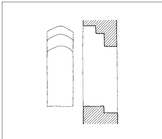
Fig. 15. Dør mellem skibets loft og tårnets mellemstokværk (s. 2409). Opstalt og snit. 1:50. Målt og tegnet af Anders C. Christensen 2016. – Door between ceiling of nave and middle floor of tower. Elevation and section.
