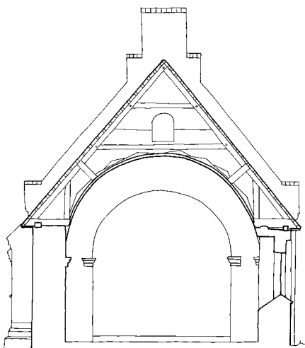
Fig. 5. Tværnsnit gennem skibet set mod øst. 1:150. Målt af Rasmus Christensen og Anders C. Christensen, tegnet af sidstnævnte 2016. – Cross-section through nave looking east.
