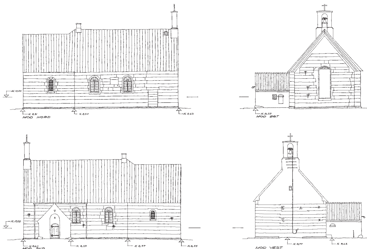
Fig. 20. Facader. 1:300. Målt af Poul Hansen og Ib Lydholm 1965. – Facades.
