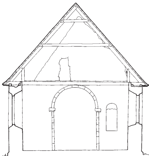
Fig. 8. Tværnsnit gennem skibet set mod øst. 1:150. Målt af Poul Hansen og Ib Lydholm 1965, suppleret og tegnet af Anders C. Christensen 2016. – Cross-section through nave looking east.
