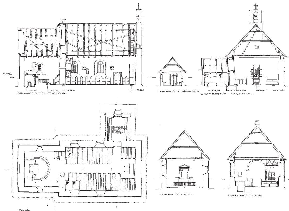
Fig. 19. Plan og snit. 1:300. Målt af Poul Hansen og Ib Lydholm 1965. – Plan and section.
