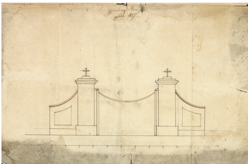
Fig. 4. Opstalt af kirkegårdsportal (s. 2479). 1:100. Tegning i RA, o. 1857. — Elevation of churchyard gate.
