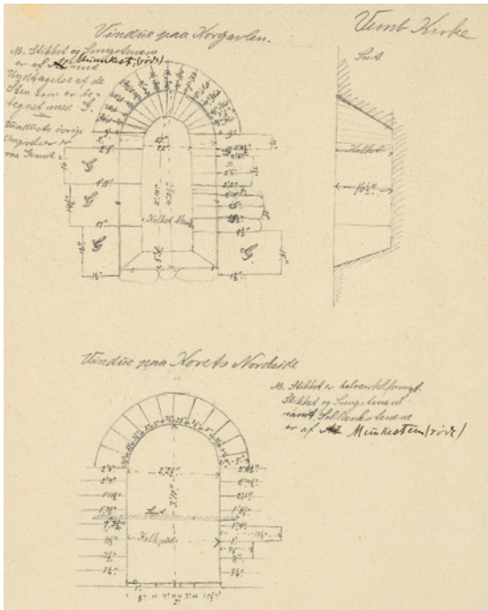
Fig. 10. Korets romanske vinduer (s. 2522). Udateret opmålingsblad ved F. Uldall. – Romanesque windows in the chancel.
