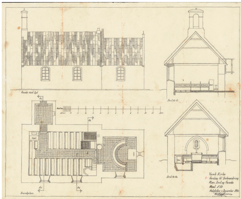
Fig. 11. Plan, snit og facader. Forslag til restaurering ved Kristian Jensen 1940 (s. 2530, 2533). 1:300. Ulfborg-Vemb Lokalhistoriske Arkiv. – Plan, section and facades. Restoration proposal by Kristian Jensen 1940.
