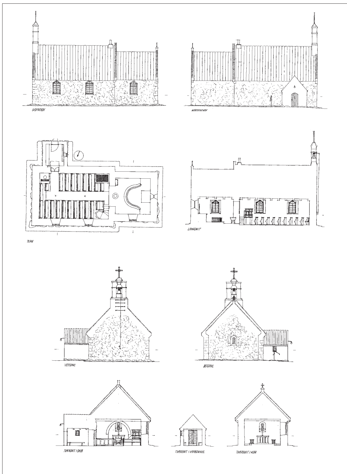
Fig. 12. Plan, snit og facader. 1.300. Målt og tegnet af Jens Foged og Poul Hansen 1958. — Plan, section and facades.
