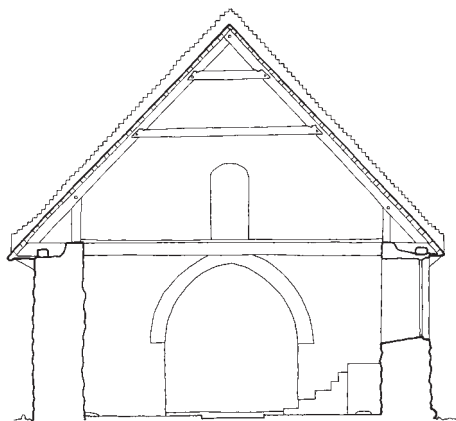
Fig. 4. Tværnsnit gennem skibet set mod øst. 1:150. Målt af Jens Foged og Poul Hansen 1958, suppleret og tegnet af Anders C. Christensen 2017. – Cross-section through the nave looking east.
