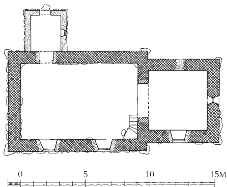
Fig. 5. Plan. 1:300. Målt af Jens Foged og Poul Hansen 1958, suppleret og tegnet af Anders C. Christensen 2017. Signaturforklaring s. 9. – Ground plan. Key on p. 9.
