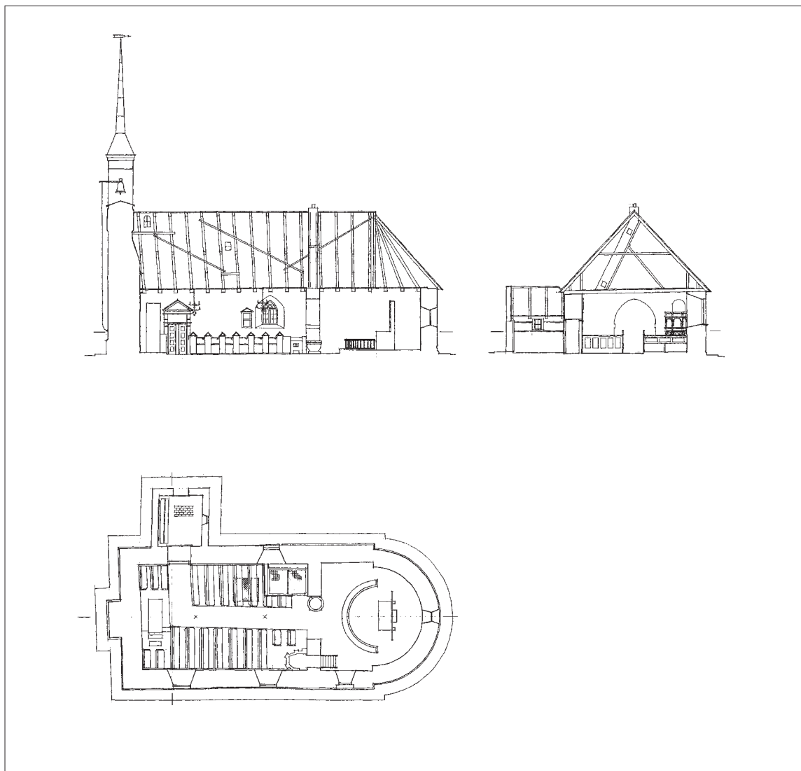
Fig. 21–22. Opstalter, snit og plan. 1:300. Målt og tegnet af Poul Hansen og Ib Lydholm 1971. – Elevations, sections and ground plan.
