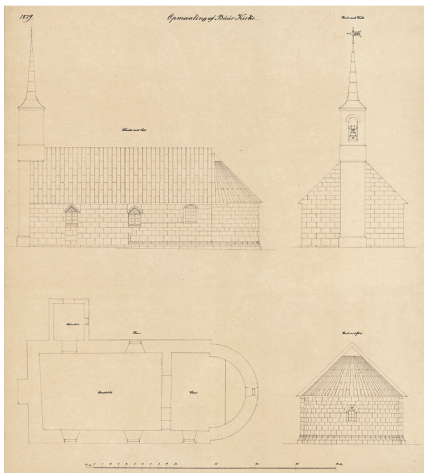
Fig. 15. Plan og facader. 1:300. Målt og tegnet af F. Uldall 1879. – Plan and facades.
