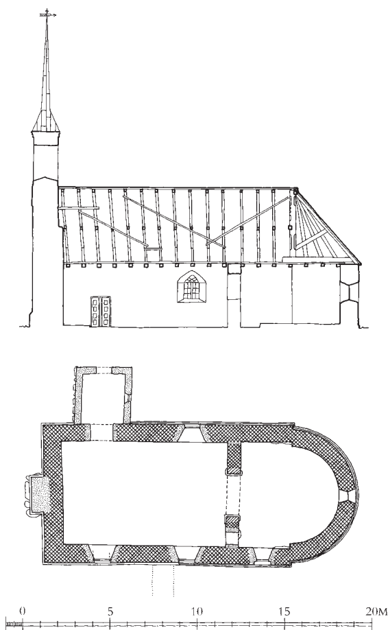
Fig. 5-6. Opmålinger. 1:300. Målt af Poul Hansen og Ib Lydholm 1971, suppleret og tegnet af Anders C. Christensen 2017. 5. Længdesnit set mod nord. 6. Plan. Signaturforklaring s. 9. – Scale drawings. 9. Longitudinal section looking north. 10. Ground plan. Key on p. 9.
