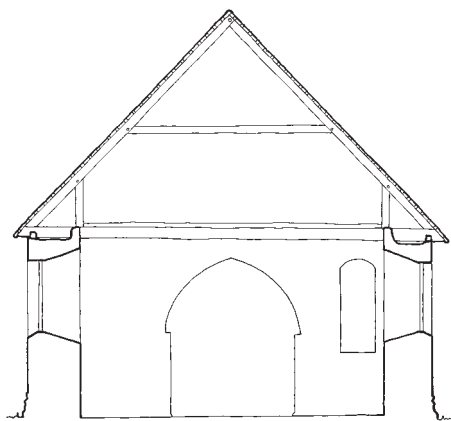
Fig. 7. Tværsnit gennem skibet set mod øst. 1:150. Målt af Poul Hansen og Ib Lydholm 1971, suppleret og tegnet af Anders C. Christensen 2017. – Cross-section through nave looking east.
