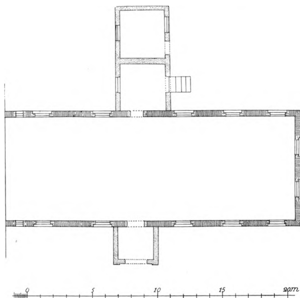
Fig. 2. Haderslev hospitalskirke. Plan. 1:300. Målt af El. M. 1951.
