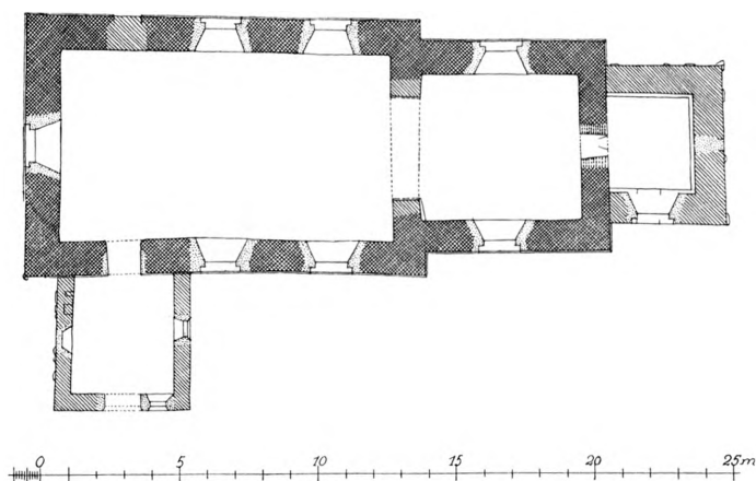
Fig. 2. Hjerndrup. Plan. 1:300. Målt af El. M. 1951.
