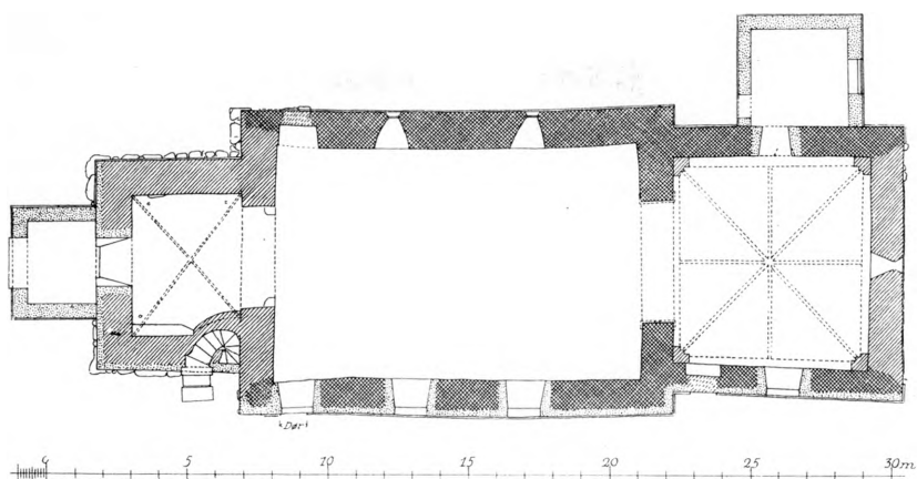
Fig. 2. Frorup. Plan. 1:300. Målt af El. M. 1951.
