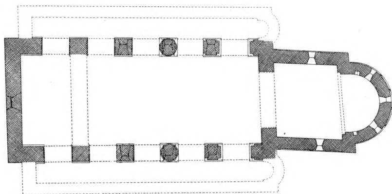
Fig. 5. Starup. Rekonstruktion af den oprindelige plan. 1:300. Ved El. M.
