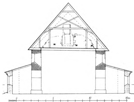
Fig. 6. Starup. Tværsnit, set mod vest. 1: 300. De punkterede linier angiver midtskibets ældste taggavl og de oprindelige sideskibsmures omtrentlige inderside.
