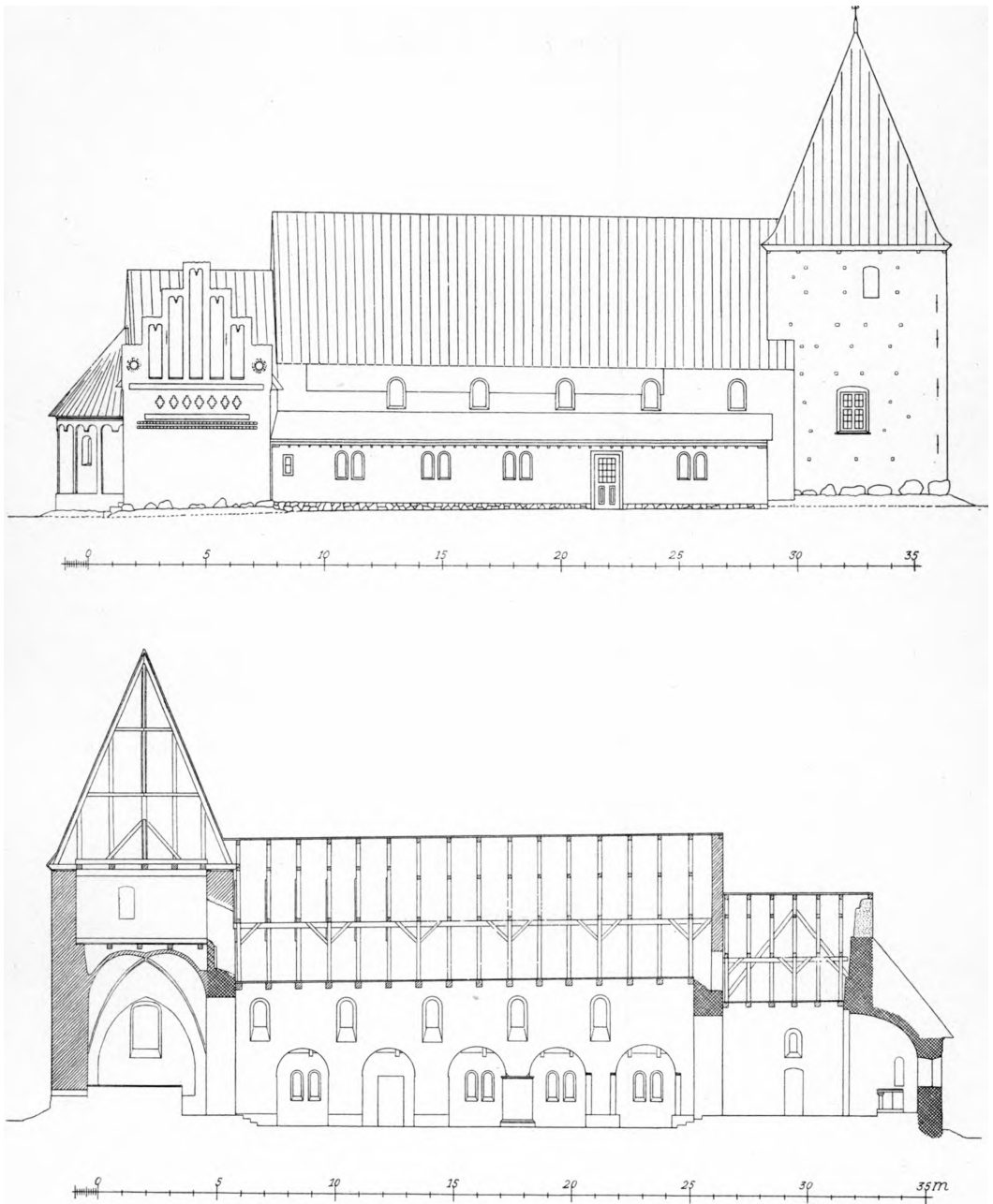
Fig. 7—8. Starup. Nordfaçade og langsnit, set mod nord. 1:300. Efter opmåling af A. Boe 1950, udlånt af V. Hardie Fischer.
