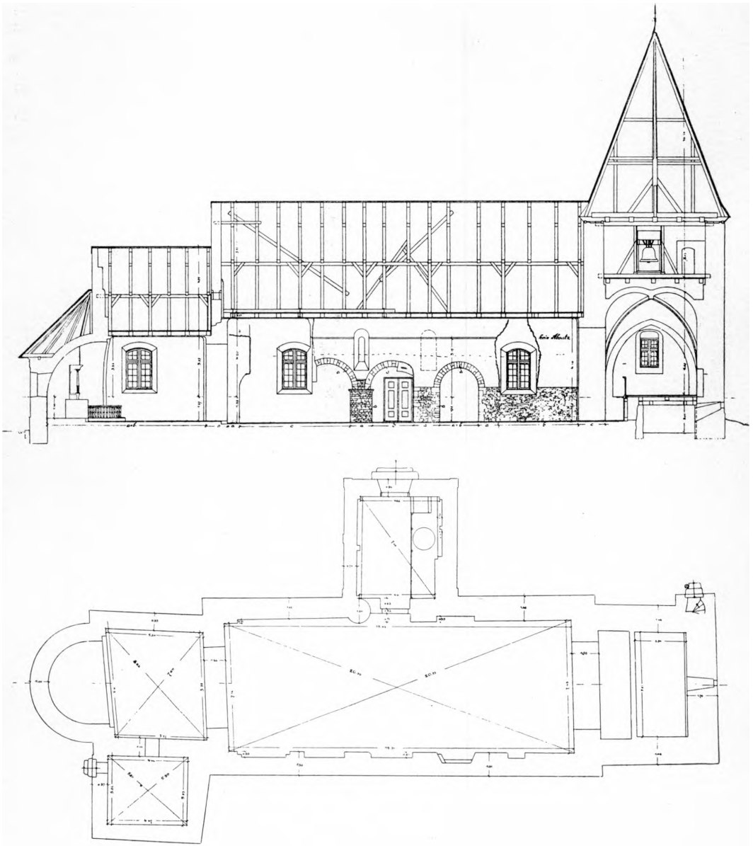
Fig. 9—10. Starup. Langsnit, set mod syd, og plan af kirken inden restaureringen. Ca. 1:300. Målt 1911 af H. Schiffmann. Opmålingen er forkert på flere punkter, bl. a. er det vandrette spring i syd-muren ført for langt vestover (sml. fig. 23).
