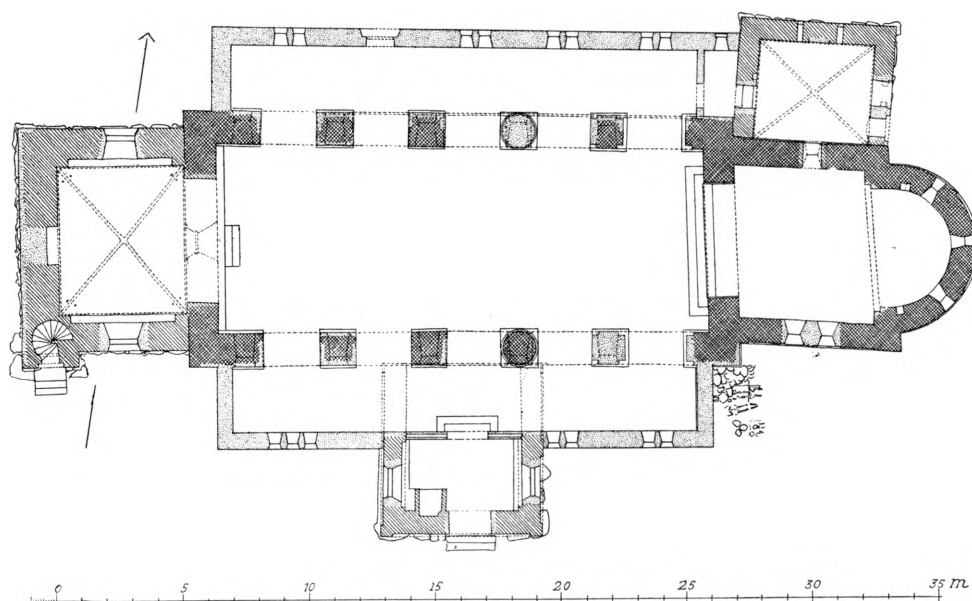
Fig. 4. Starup. Plan. 1:300. Målt af Erik Hansen. 1952.
