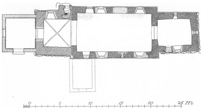
Fig. 2. Skrave. Plan. 1:300. Målt af Erik Hansen 1952.
