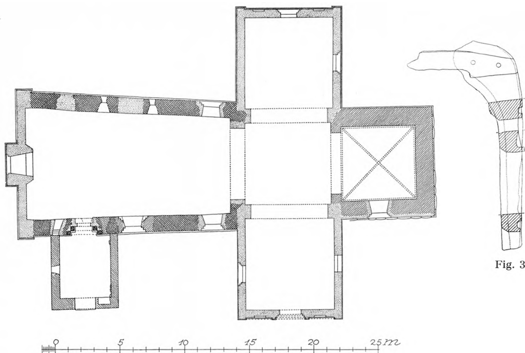
Fig. 2. Skodbore. Plan. 1:300. Målt af Erik Hansen 1952.
