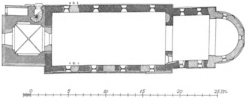
Fig. 2. Lintrup. Plan. 1:300. Målt af El. M. 1952.
