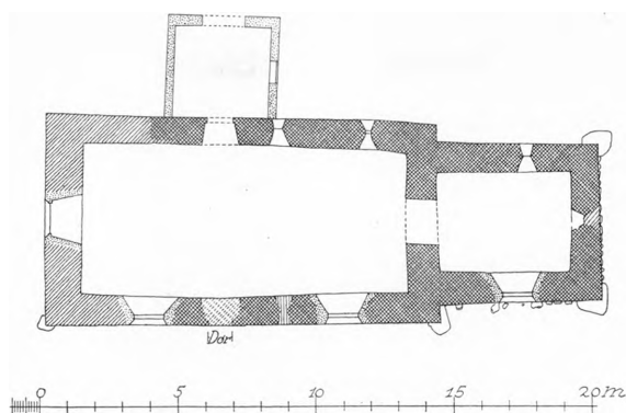
Fig. 2. Hjerting. Plan. 1:300. Målt af El. M. 1952.
