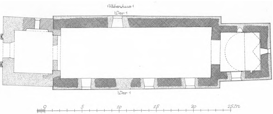
Fig. 2. Fole. Plan. 1:300. Målt af El. M. 1952.
