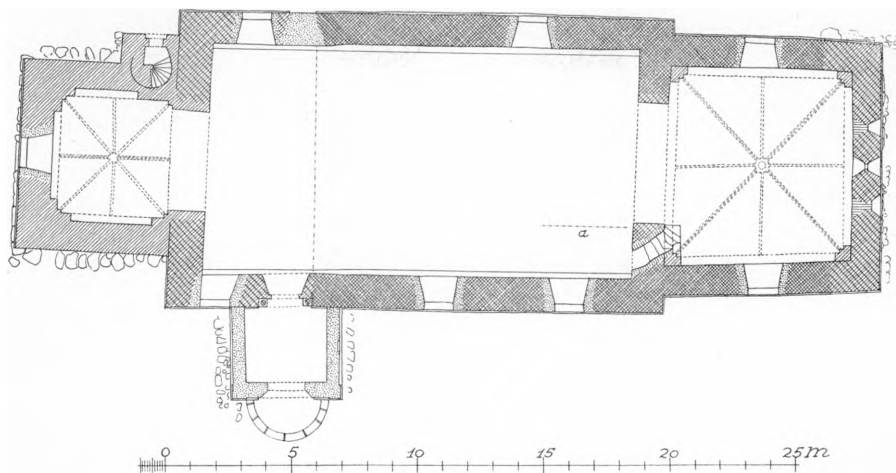
Fig. 2. Bevtøft. Plan. 1:300. Målt af El. M. 1953. Den stiplede linje, a, markerer det oprindelige kapels omtrentlige udstrækning mod syd (p. 889).
