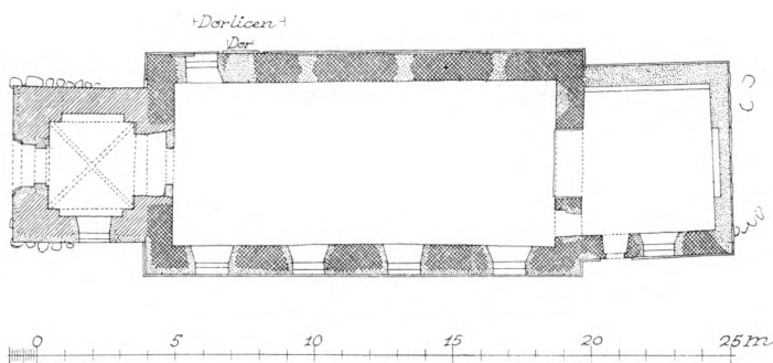
Fig. 2. Højrup. Plan. 1:300. Målt af El. M. 1953.
