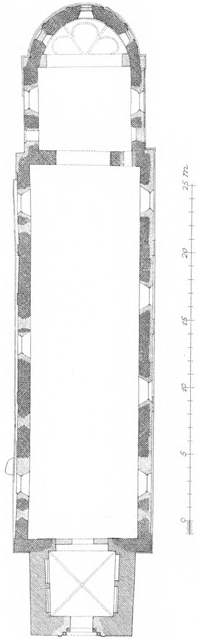
Fig. 5. Brøns. Plan. 1: 300. Øst opad. Målt af Erik Hansen 1953.
