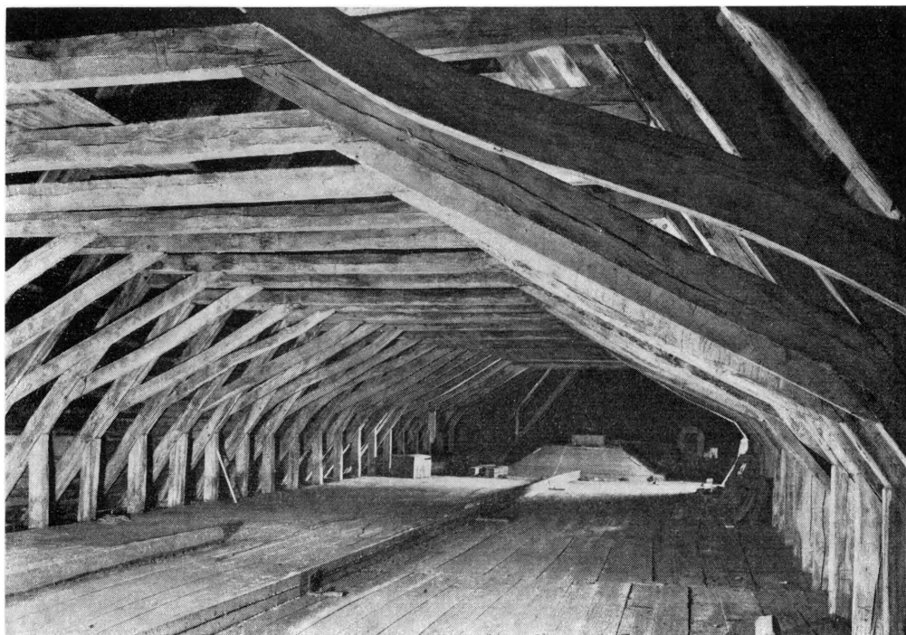
Fig. 7. Brønshøj. Skibets tagværk, set mod vest (p. 1222).
