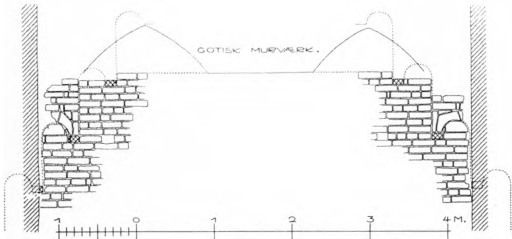
Fig. 3. Brøns. Skibets vestgavl. 1:100. Målt af Erik Hansen 1953 (p. 1220).
