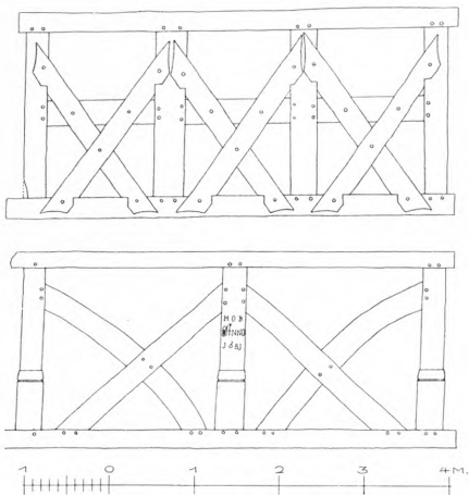
Fig. 4. Brøns. Klokkestol. 1:100. Målt af El. M. 1953 (p. 1238).
