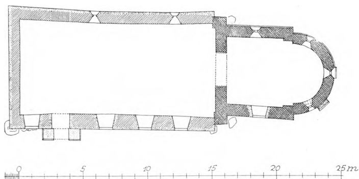
Fig. 2. Ubjærg. Plan. 1:300. Målt af El. M. 1954.
