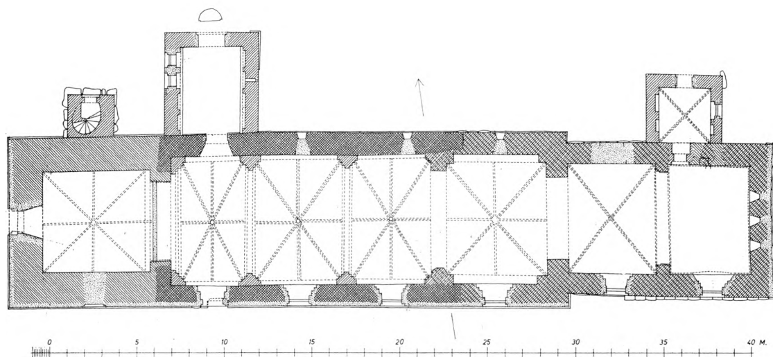
Fig. 2. Emmerlev. Plan. 1:300. Målt af El. M. 1955.
