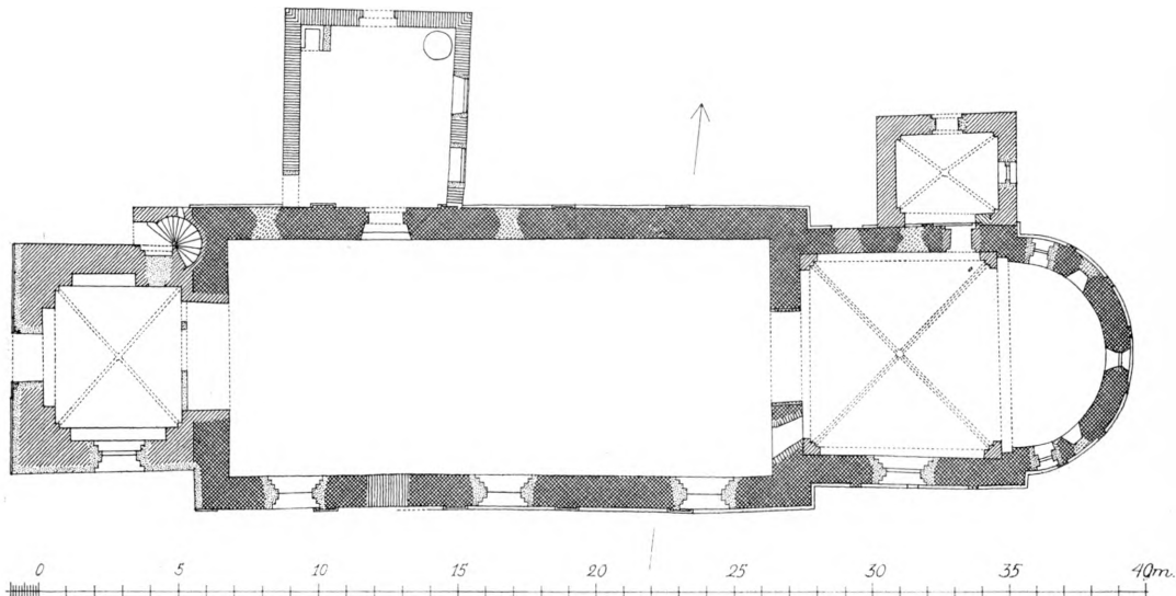
Fig. 2. Ballum. Plan 1:300. Målt af John Petersen 1956.
