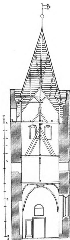
Fig. 3. Ballum. Tårn. Snit, set mod øst. 1:300. Målt af Mette Pihler 1956 (p. 1405).
