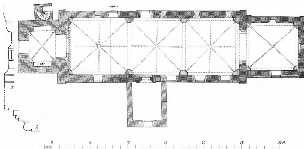
Fig. 2. Nørre-Løgum. Plan. 1:300. Målt af El. M. 1955 samt til venstre (a) snit gennem øvre del af dørfremspringet i syd og (b) dørens yderprofil. 1: 30 (p. 1526).
