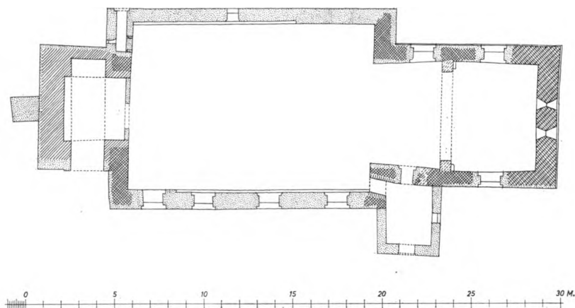
Fig. 2. Abild. Plan. 1:300. Målt af El. M. 1954.
