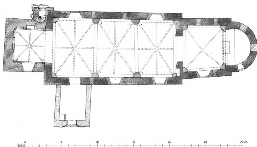
Fig. 2. Højst. Plan. 1:300. Målt af El. M. 1954.
